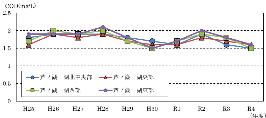
図2 湖沼の環境基準非達成地点におけるCOD年間平均値の推移
