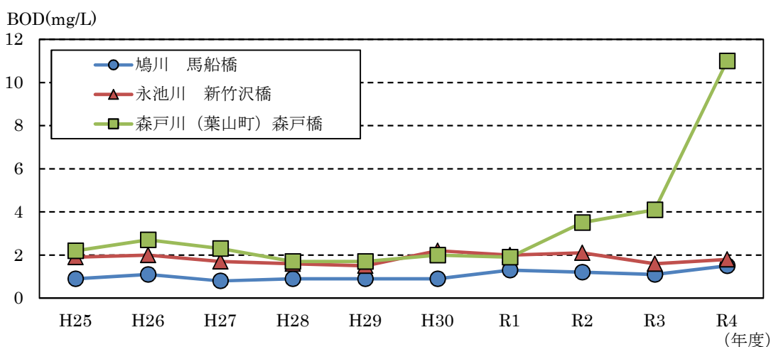
図1 河川的环境基準非達成地点におけるBOD年間平均値の推移
