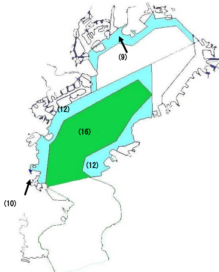
図4 東京湾におけるCODの環境基準非達成水域
