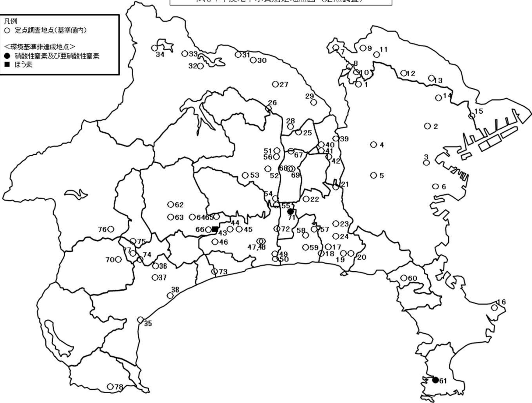
令和4年度地下水質測定地点図（定点調査）
