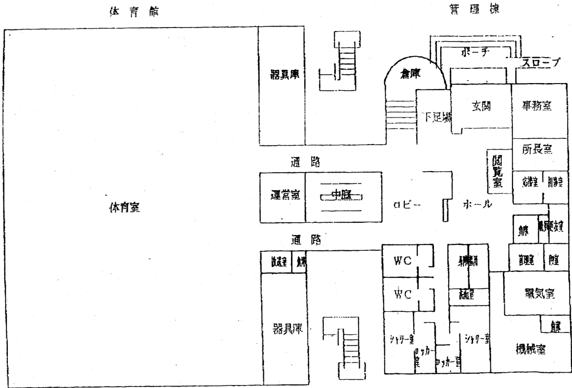
センター平面図 1F
