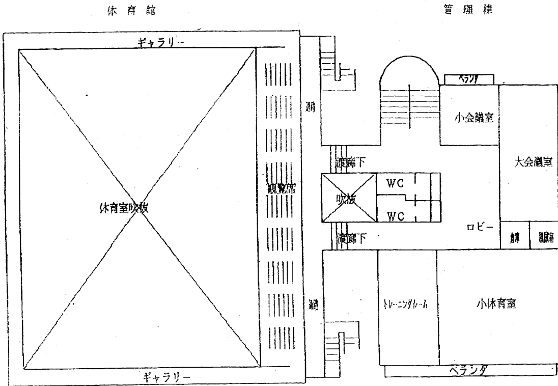
センター平面図 2F
