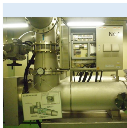
【紫外線処理設備（県企業庁）】
