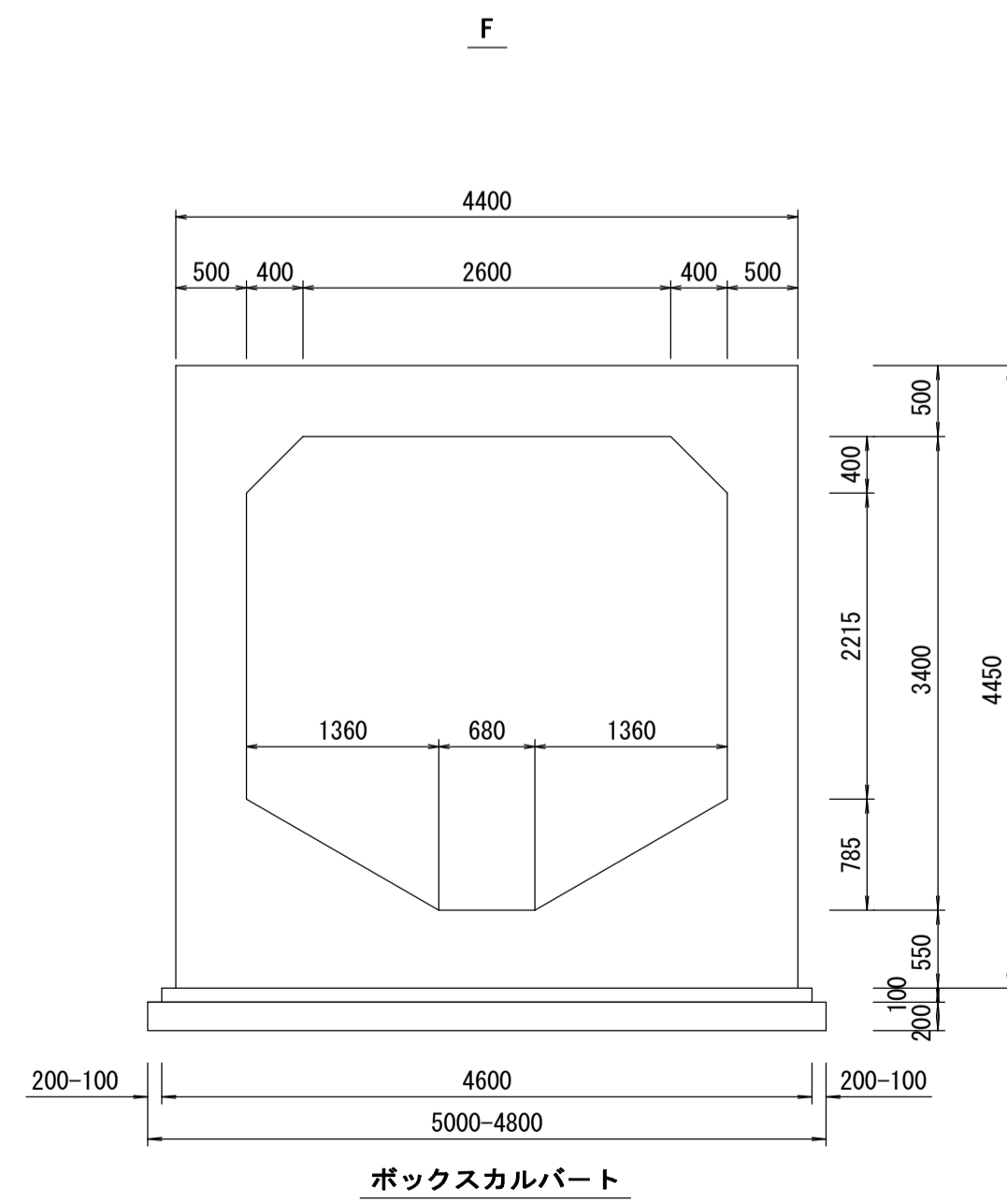
管渠構造図 S=1:50
