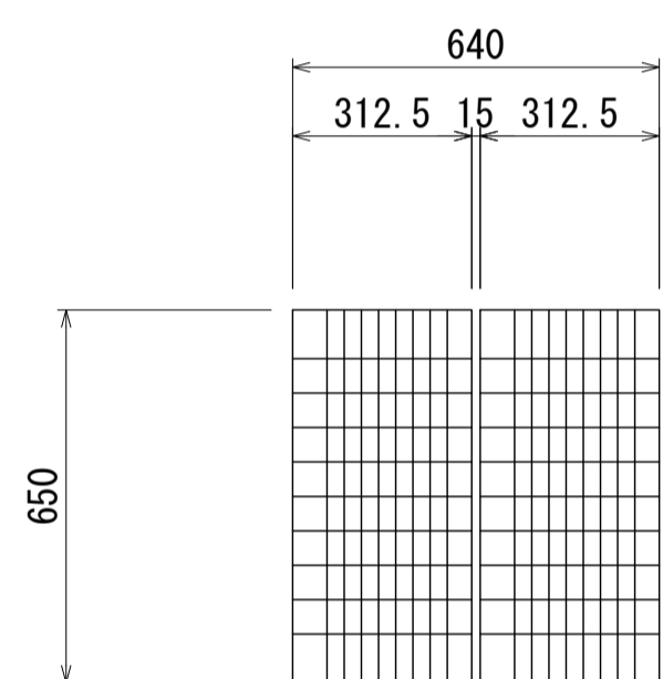
グレーチング受枠 S=1:15
