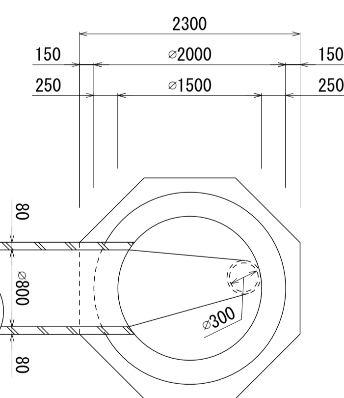
C - C 断面図 S=1:40
