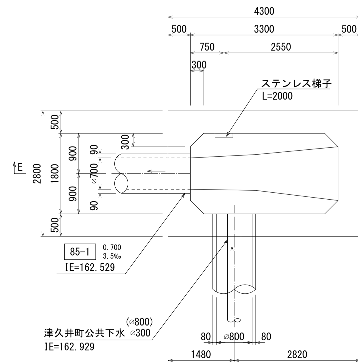
D - D 断面図 S=1:50
