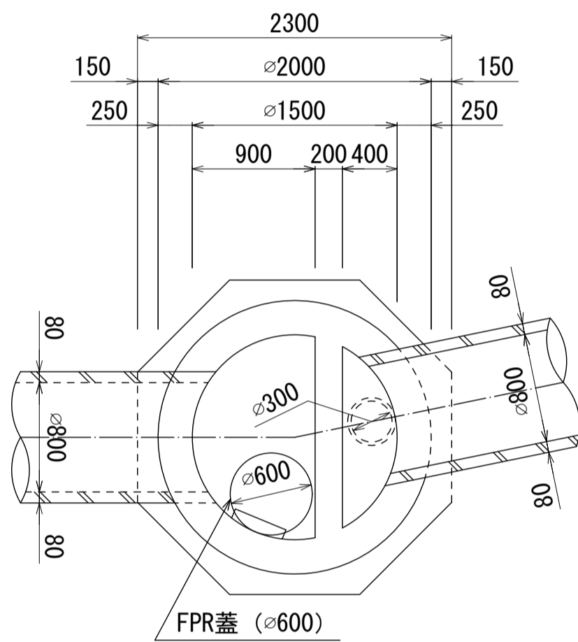
B - B 断面図 S=1:40
