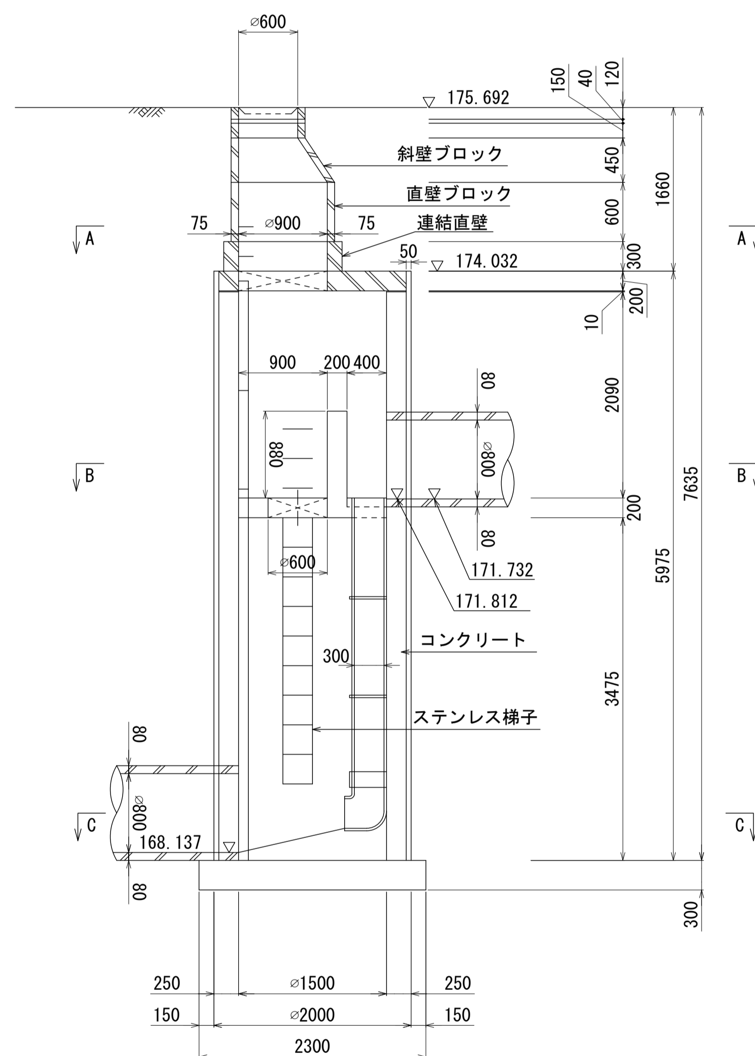
D - D 断面図 S=1:40
