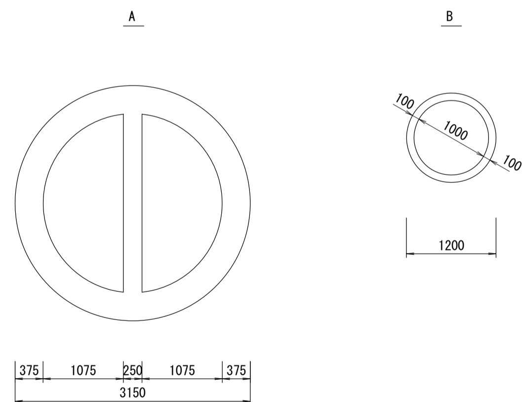
管渠構造図 S=1:50
