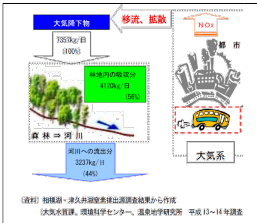
<図 窒素の移流・拡散・流出のメカニズム>
