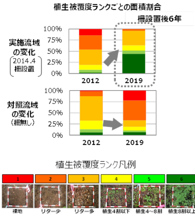
<図 小流域スケールの下層植生変化>
