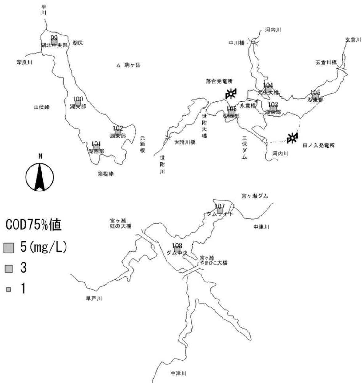
図 2 - 2 湖沼の汚濁状況図（上段左：芦ノ湖、上段右：丹沢湖、下段：宮ヶ瀬湖） (COD75%値)
