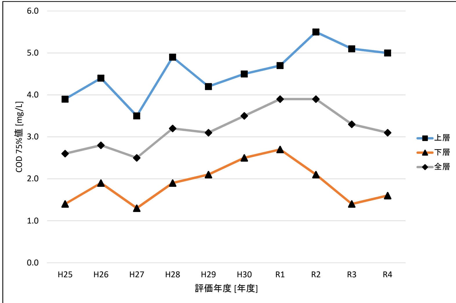
図7-7 東京湾・扇島沖におけるCOD75%値の経年推移
