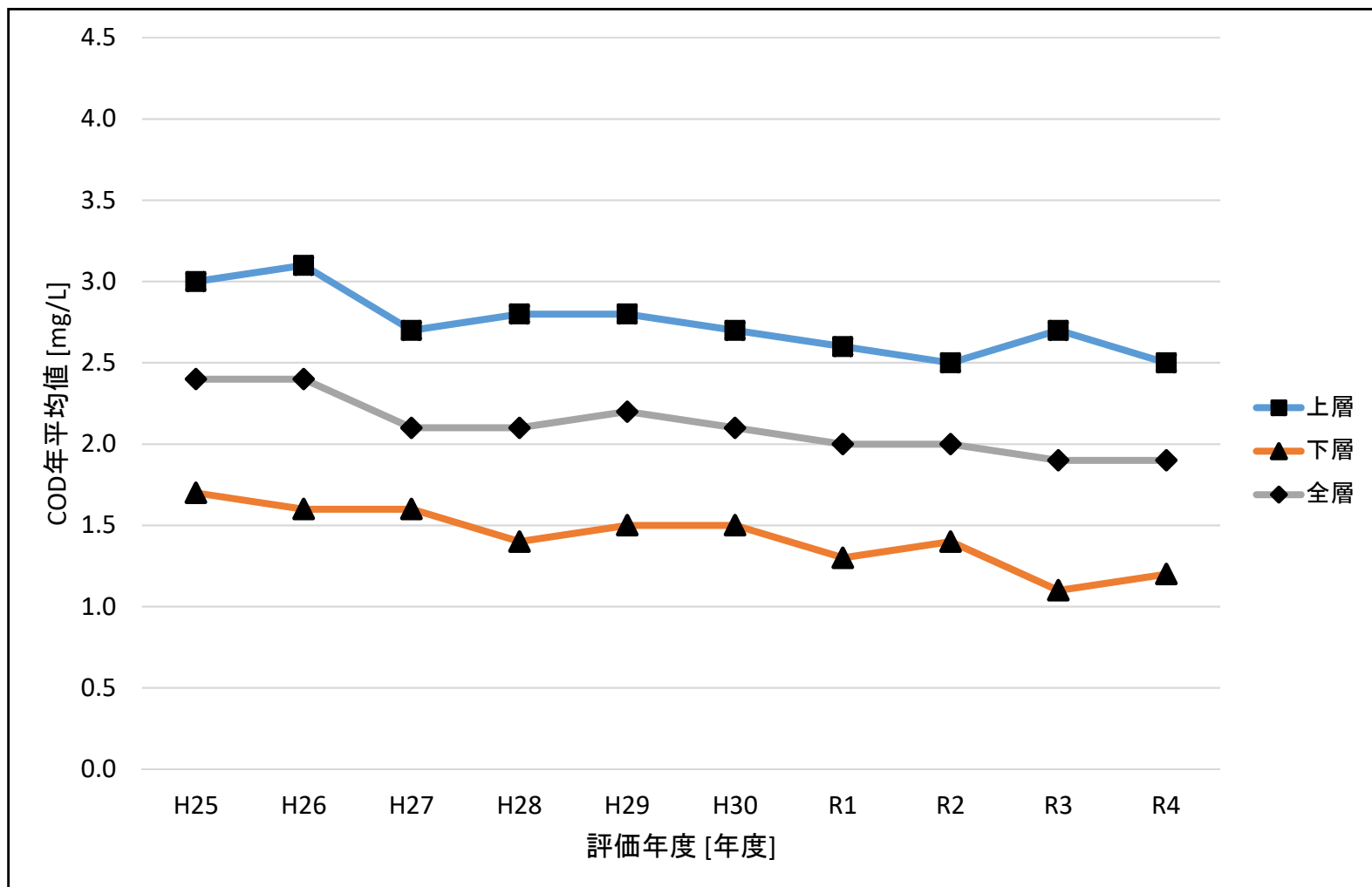
図7-12 東京湾・中の瀬南におけるCOD年平均値の経年推移
