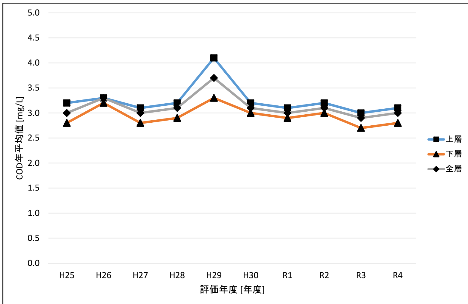
図7-4 東京湾・平潟湾内におけるCOD年平均値の経年推移
