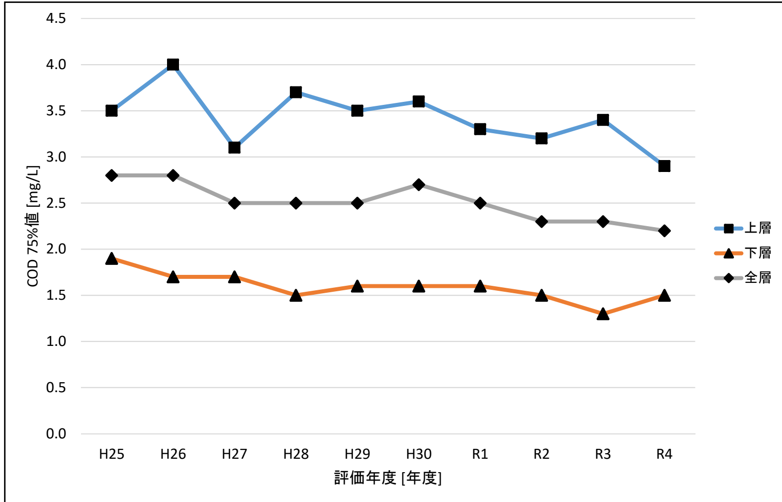
図7-11 東京湾・中の瀬南におけるCOD75%値の経年推移
