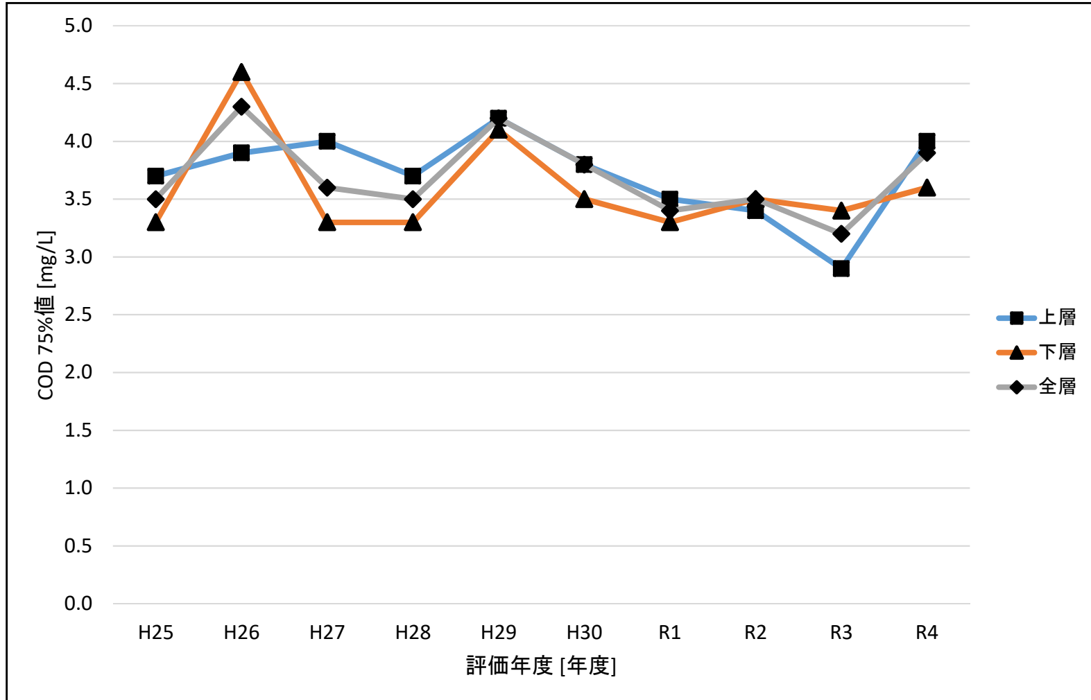
図7-3 東京湾・平潟湾内におけるCOD75%値の経年推移
