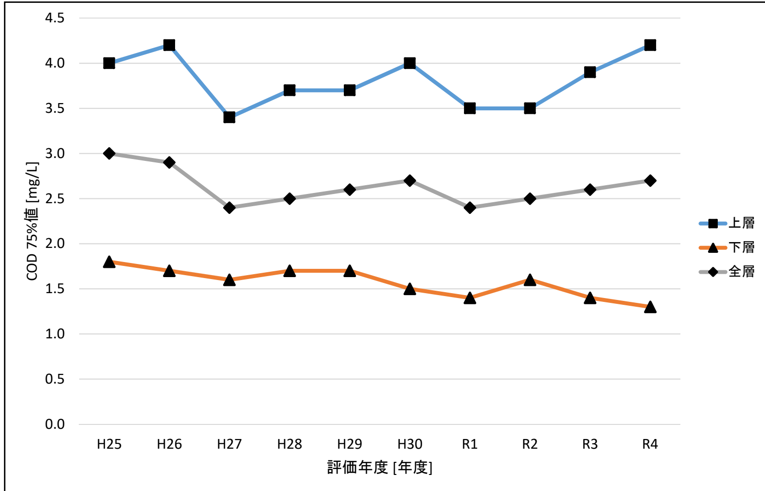
図7-9 東京湾・中の瀬北におけるCOD75%値の経年推移
