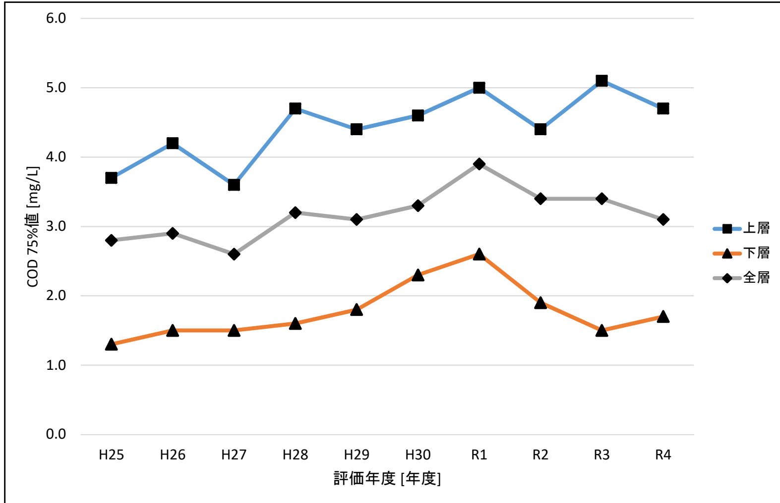
図7-5 東京湾・東扇島沖におけるCOD75%値の経年推移
