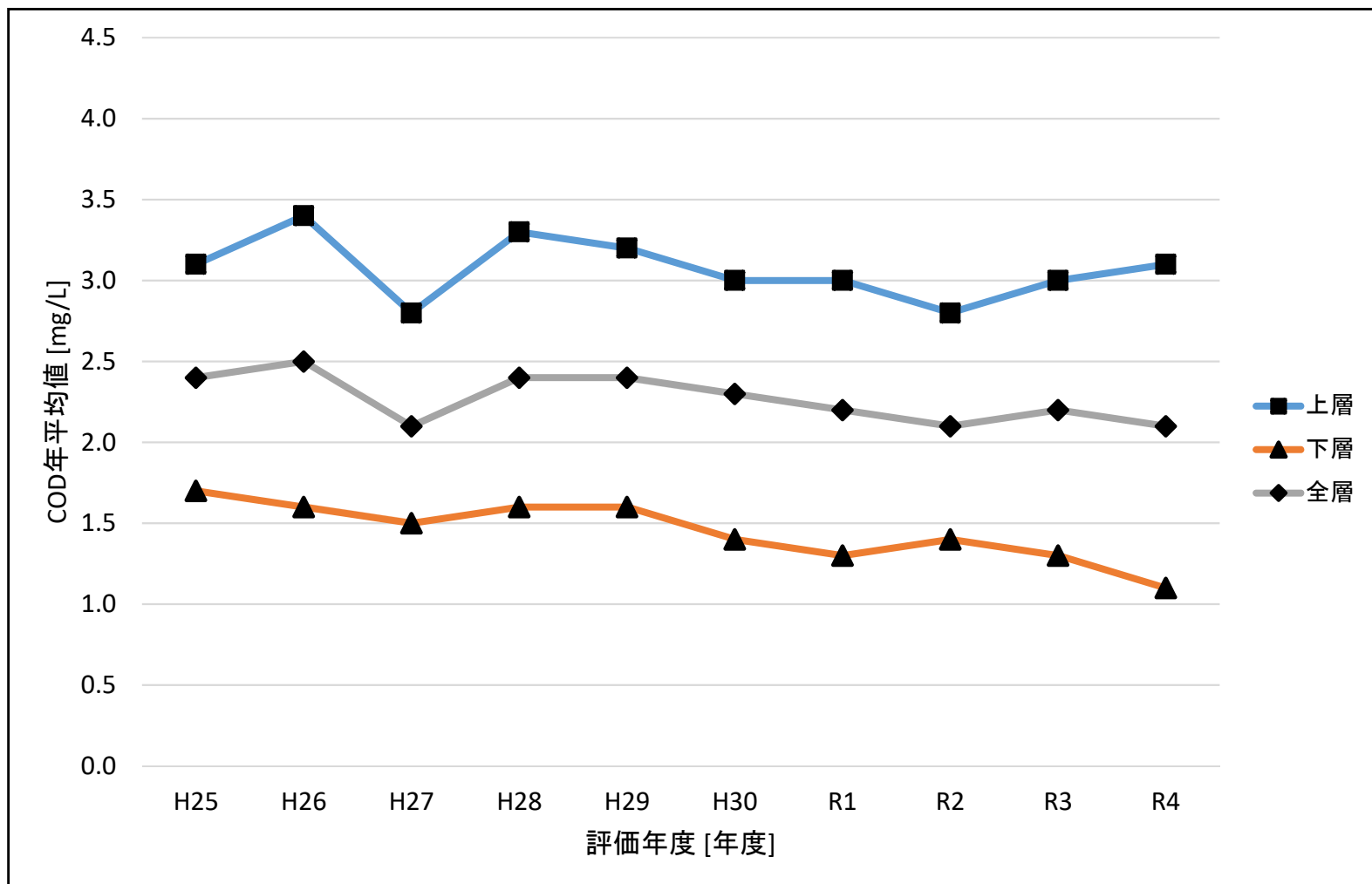
図7-10 東京湾・中の瀬北におけるCOD年平均値の経年推移
