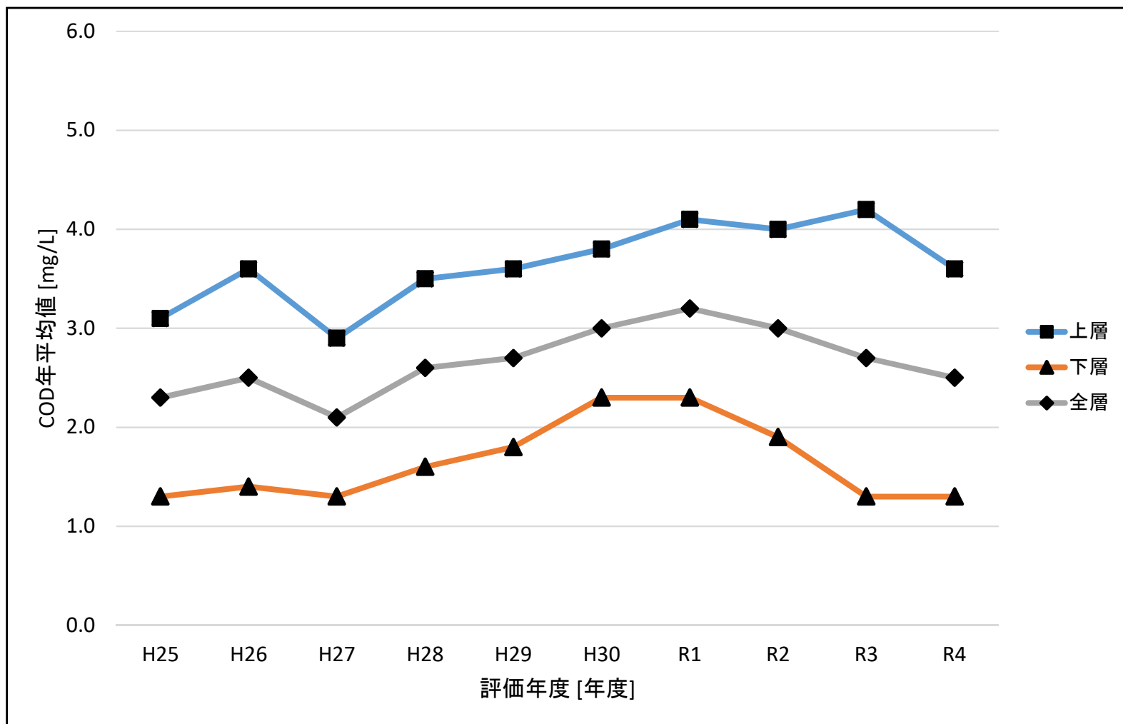
図7-8 東京湾・扇島沖におけるCOD年平均値の経年推移
