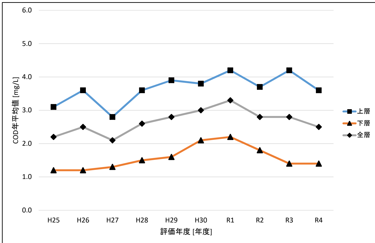
図7-6 東京湾・東扇島沖におけるCOD年平均値の経年推移
