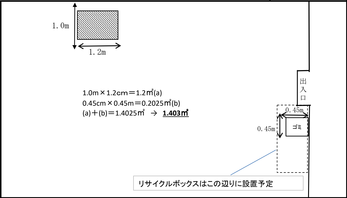
配 置 図
