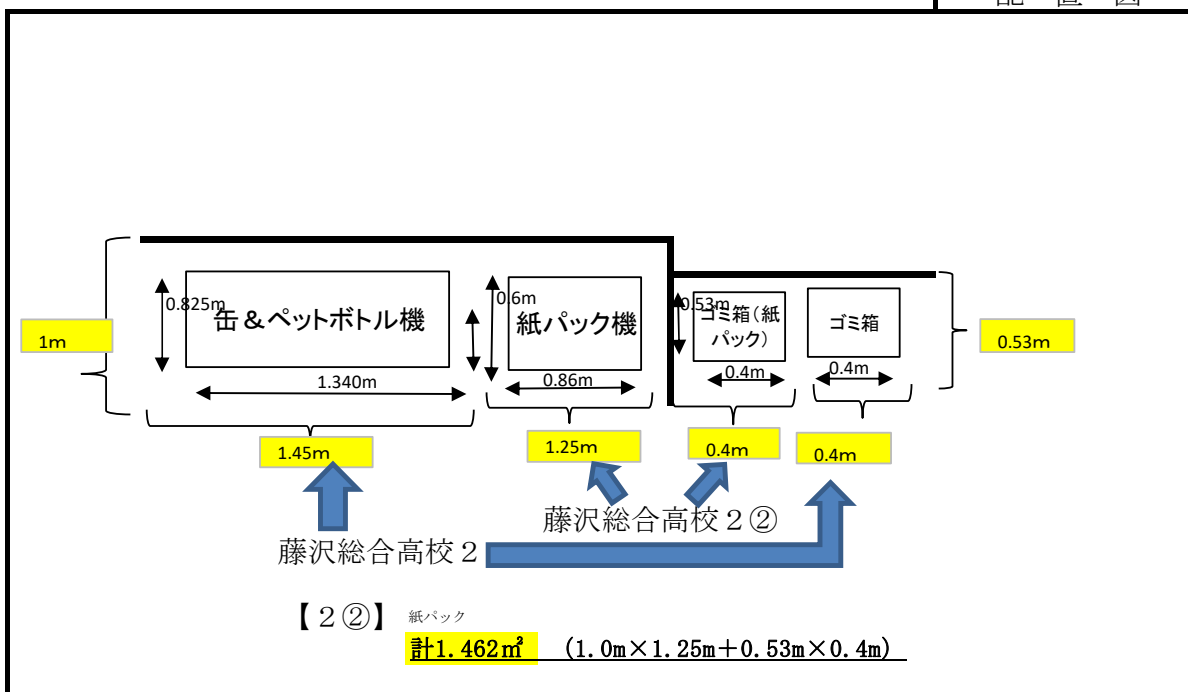
配置図
