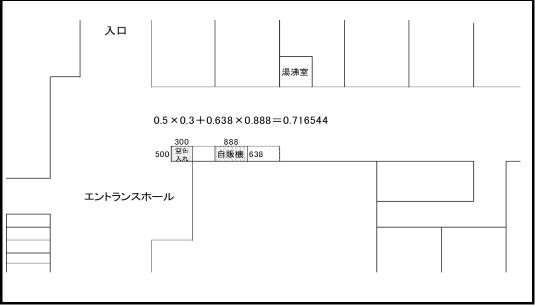
配置図
