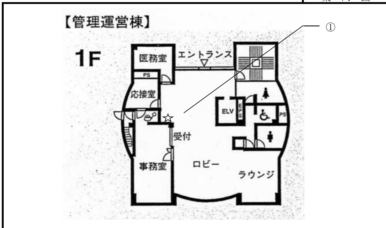
案内図
