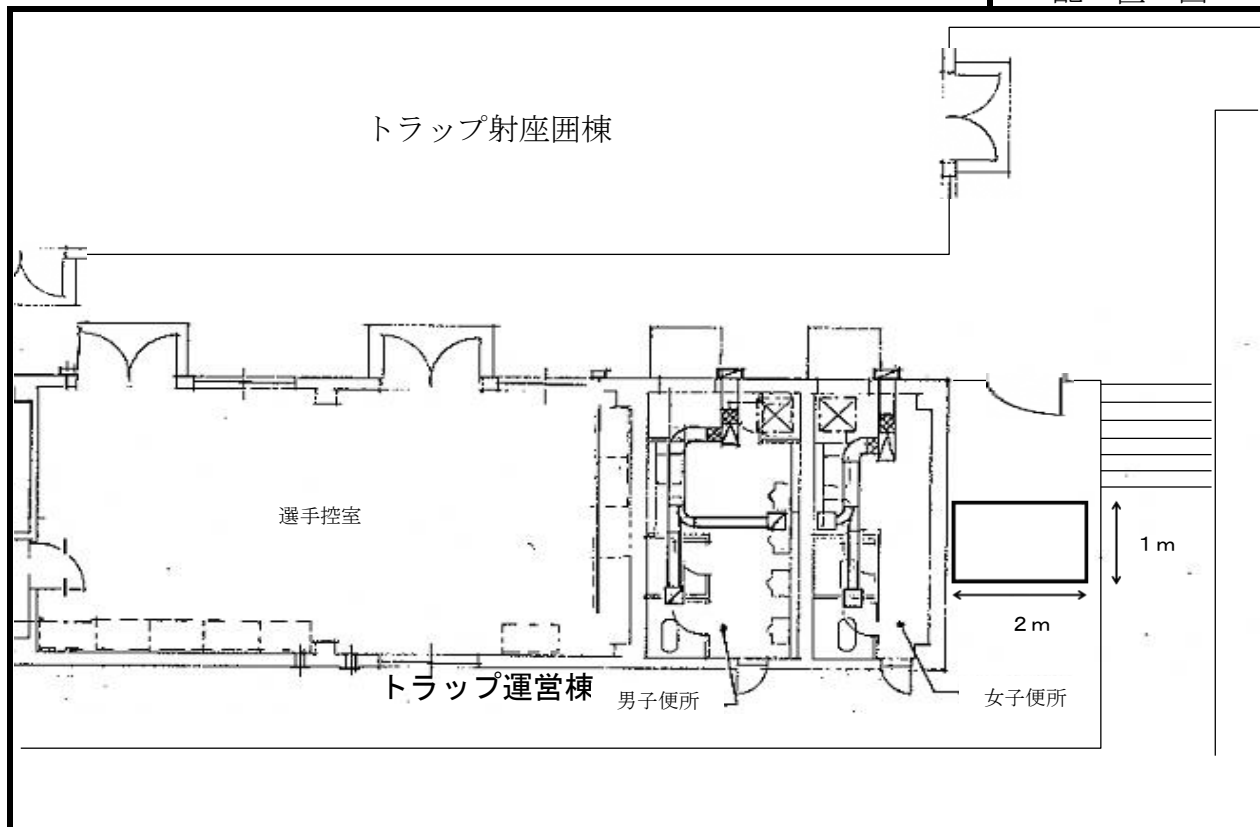
配置図
