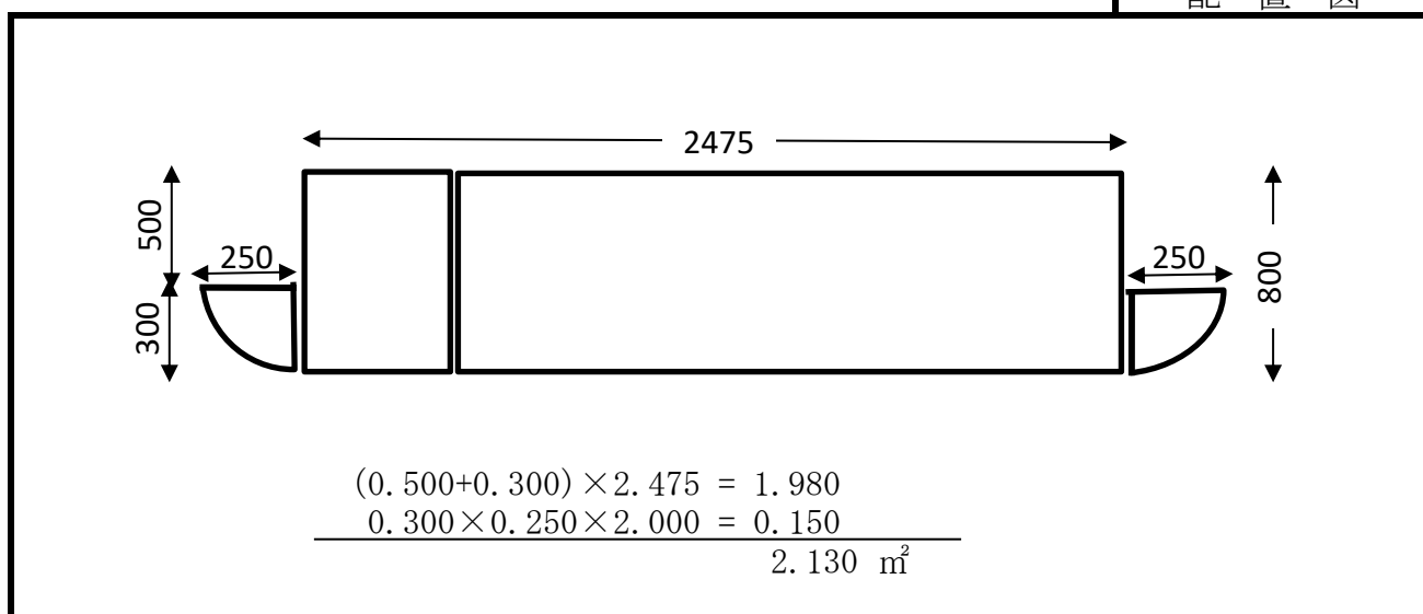
配置図
