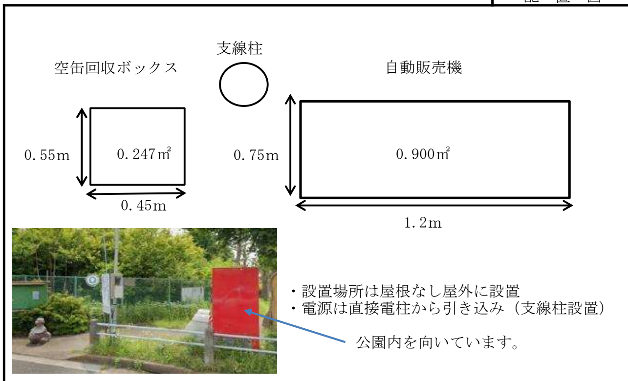
配置図
