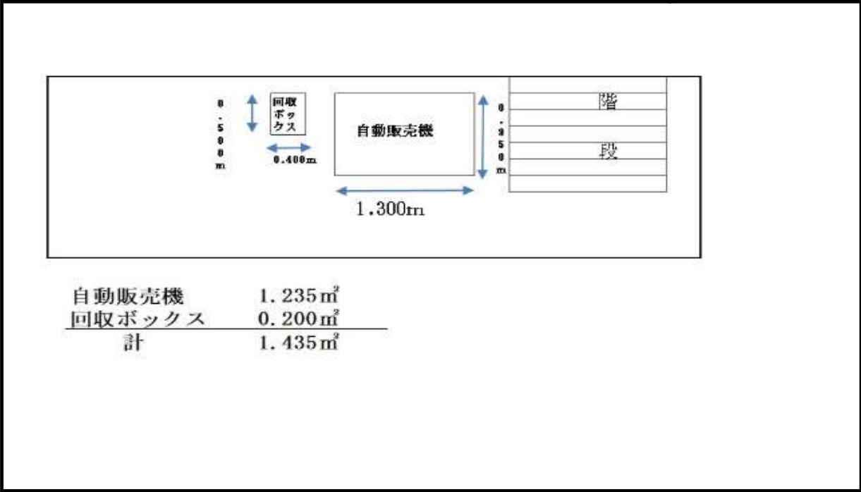
配置図
