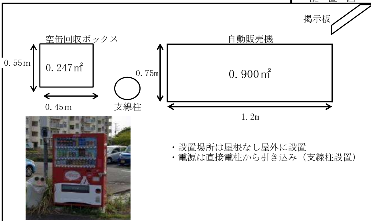
配置図
