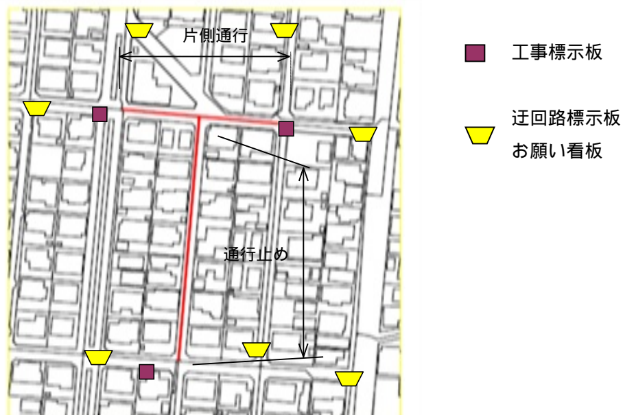
交通規制計画図，保安施設設置計画
