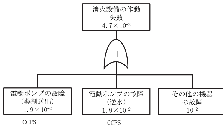
図 4.2.3 消火設備の作動失敗に関する FTA（平常時）
