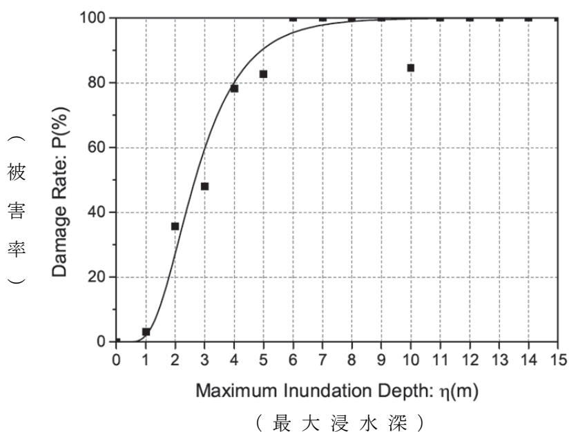
図 8.3.1 2011 年東北地方太平洋沖地震の際の石油タンク付属配管 津波被害率 (■) と被害率曲線 (実線) i
