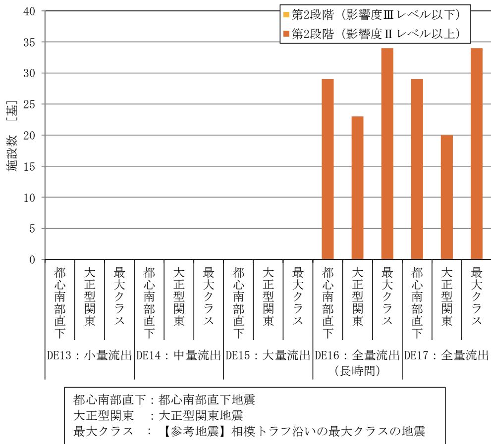
図 5.5.7(2) 京浜臨海地区における第2段階の災害に該当する施設数の比較 (高圧ガスタンク・毒性ガス拡散)
