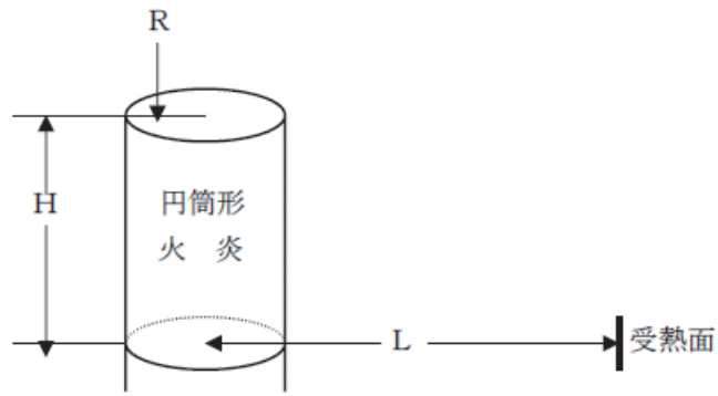
図 3.1 円筒形火炎と受熱面の位置関係
