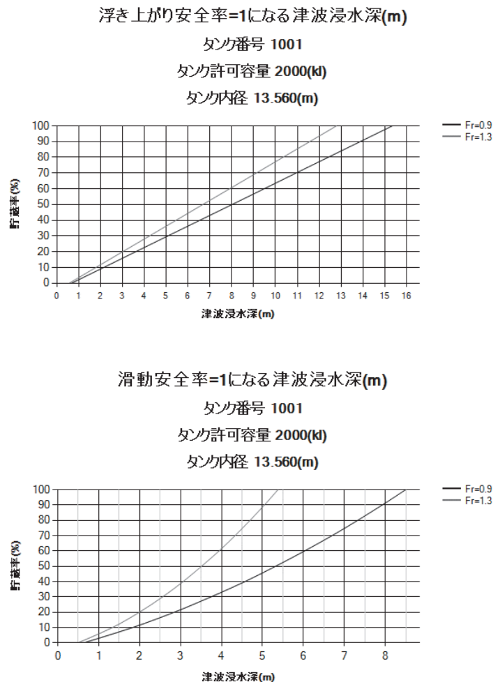
図 8.3.2 津波被害シミュレーション結果の一例 (上図：浮き上がり安全率，下図：滑動安全率)
