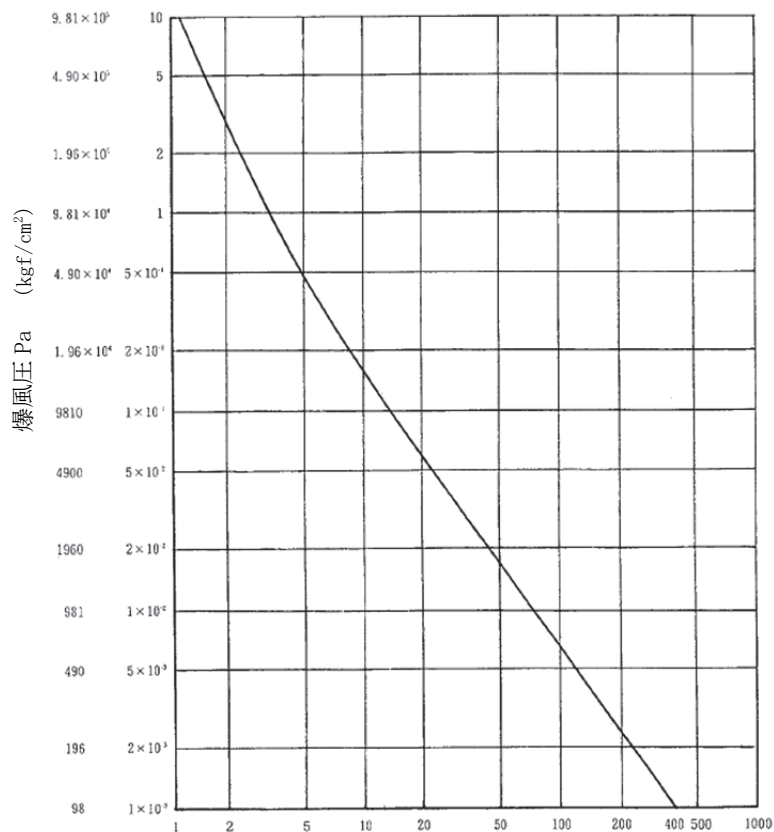
図 3.6 換算距離 \lambda と爆風圧との関係 ii
