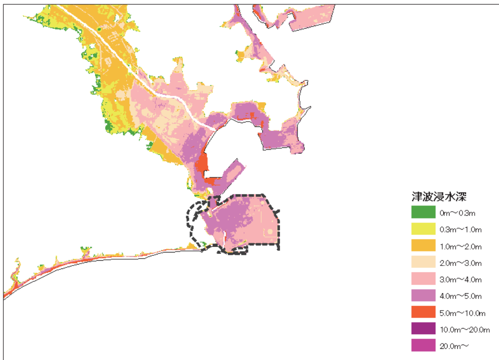
図 8. 2. 2(3) 【参考地震】相模トラフ沿いの最大クラスの地震（西側モデル） における津波浸水予測図（久里浜地区）
