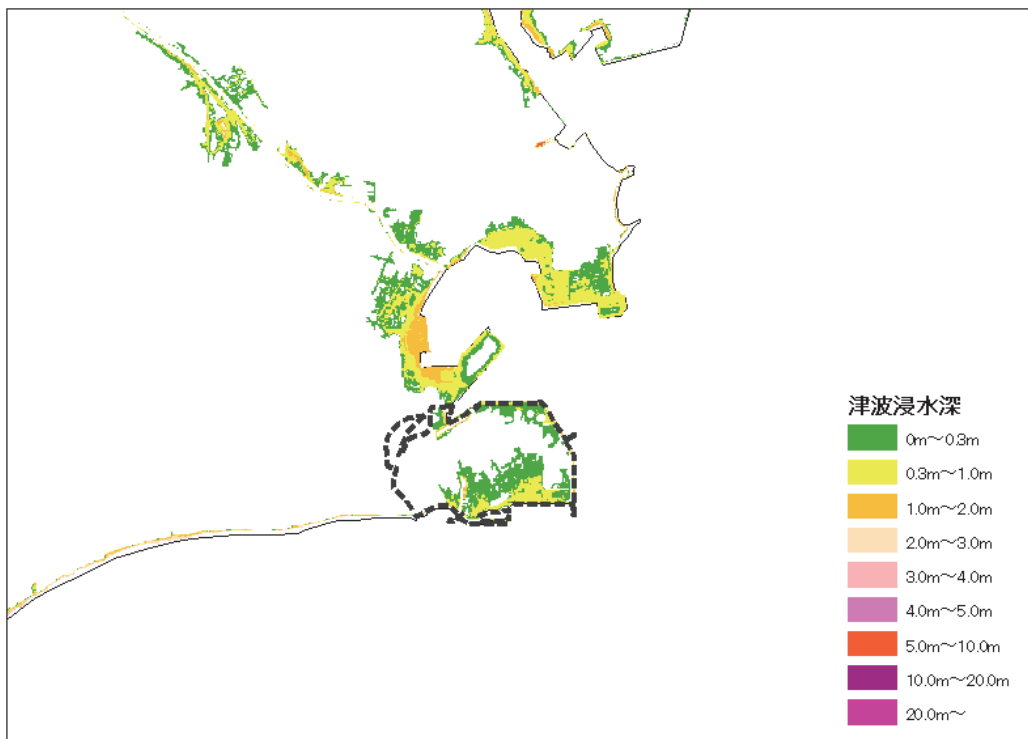
図 8. 2. 1 (3) 大正型関東地震における津波浸水予測図 (久里浜地区)
