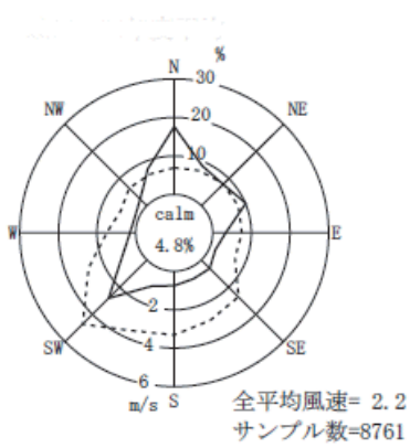
図 4.4 風配図 (中区本牧, 過去5年間の平均)
