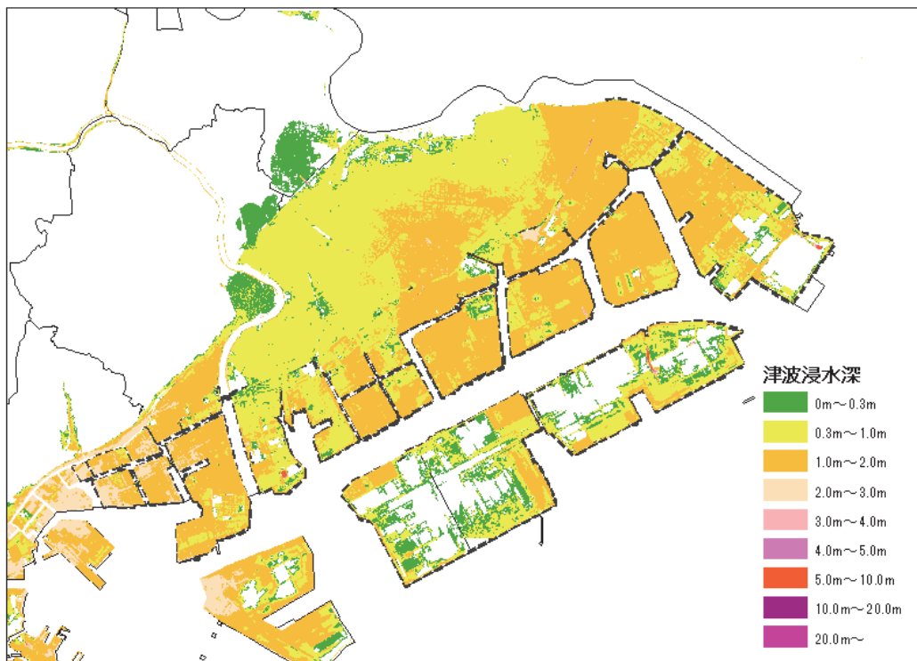
図 8.2.2(1) 【参考地震】相模トラフ沿いの最大クラスの地震（中央モデル） における津波浸水予測図（京浜臨海地区）
