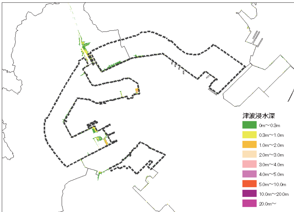
図 8. 2. 1 (2) 南海トラフ巨大地震における津波浸水予測図 (根岸臨海地区)
