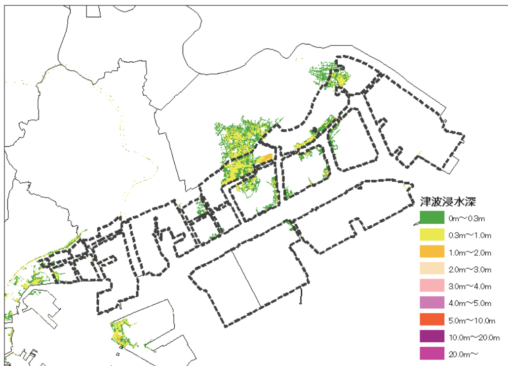
図 8. 2. 1 (1) 南海トラフ巨大地震における津波浸水予測図 (京浜臨海地区)
