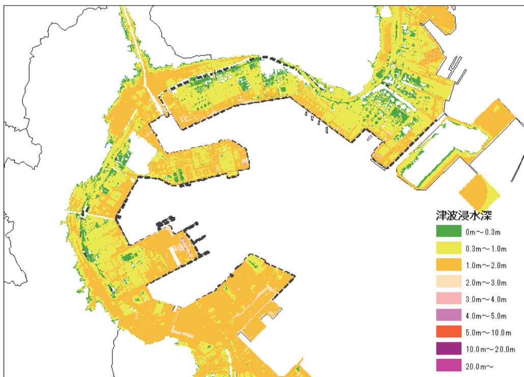
図 8.2.2(2) 【参考地震】相模トラフ沿いの最大クラスの地震（中央モデル） における津波浸水予測図（根岸臨海地区）
