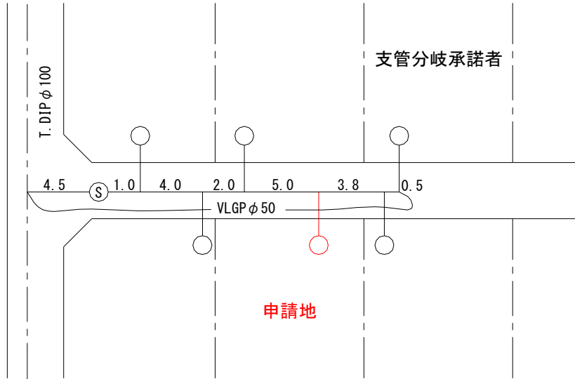
図4-2-7 平面図
