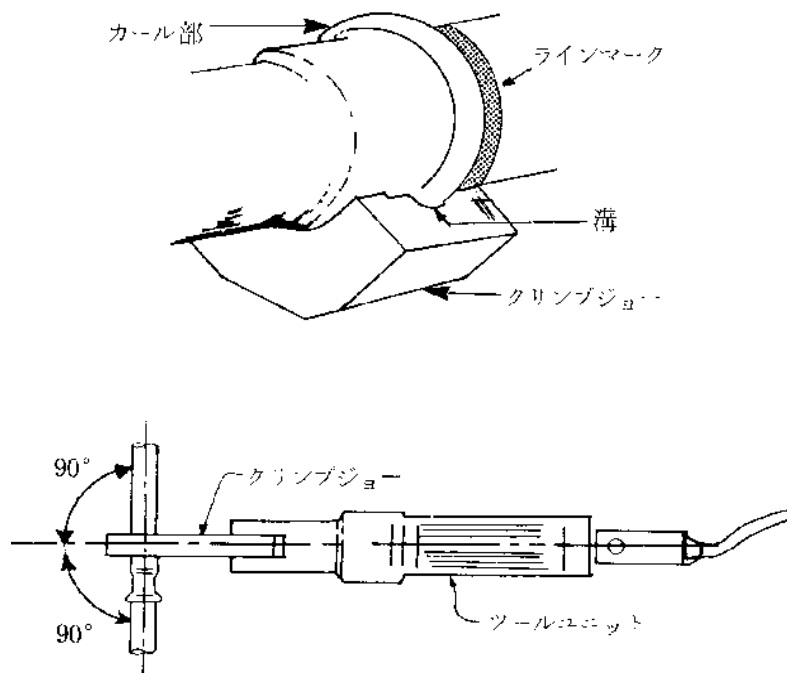
図5-6-12 プレス式
