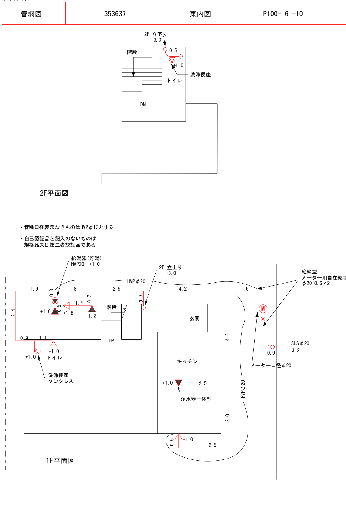
図4-2-1-1 平面図
