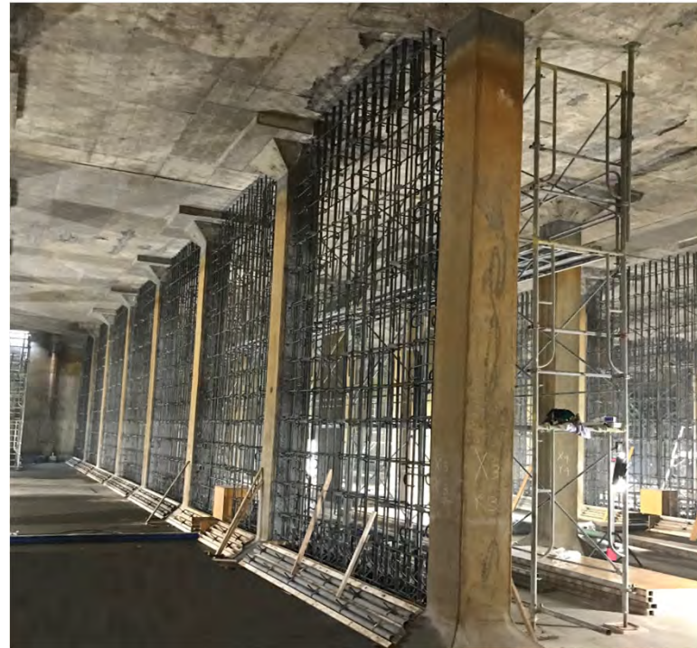
二本松配水池（藤沢市）内部に新たに強度のある壁を施工している様子
