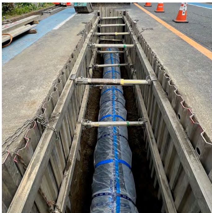
茅ヶ崎市赤羽根～東海岸基幹管路 更新工事 耐震継手管埋設工の様子
