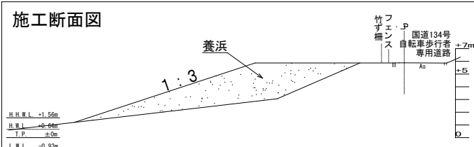
将来断面図
