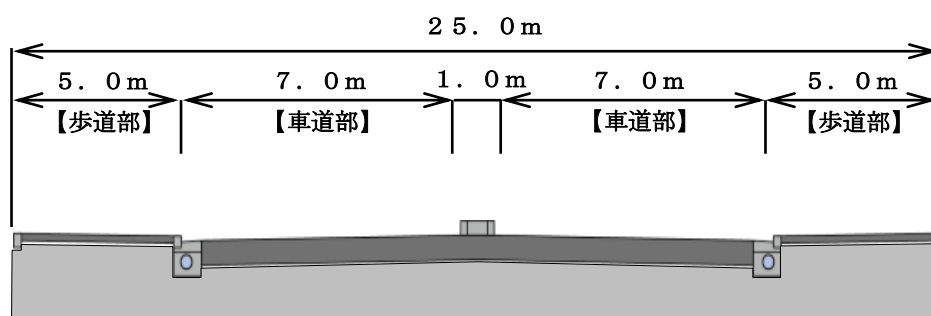
（標準横断図）
