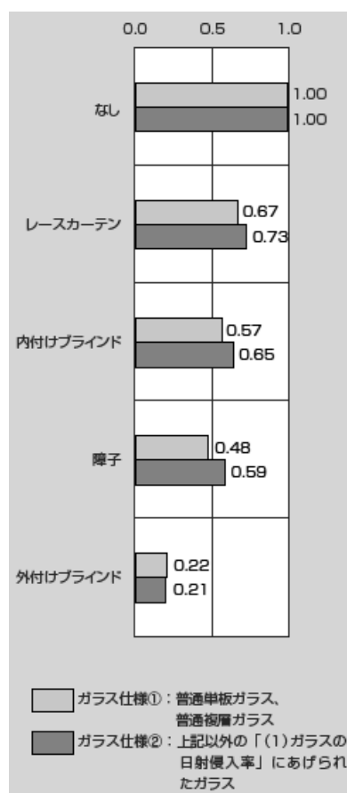
図 1.3.5 日射遮へい部材の日射遮へい係数
