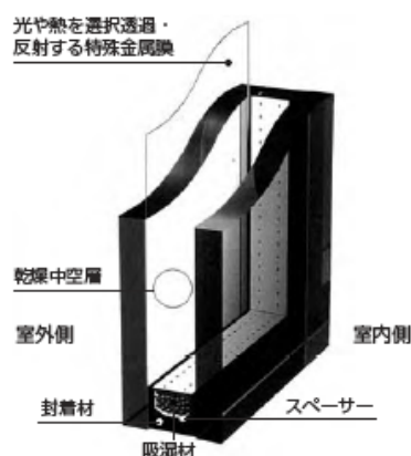
図 1.3.3 遮熱型低放射率複層ガラス
