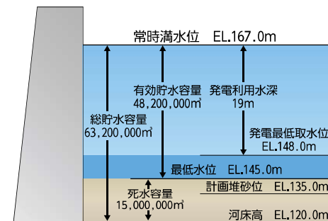
相模ダム容量配分図
