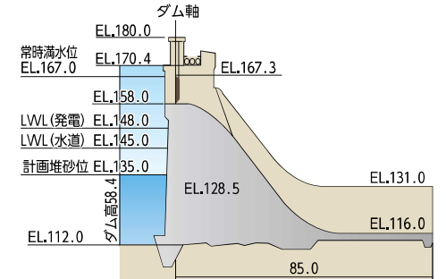
相模ダム標準断面図 (単位:メートル)
