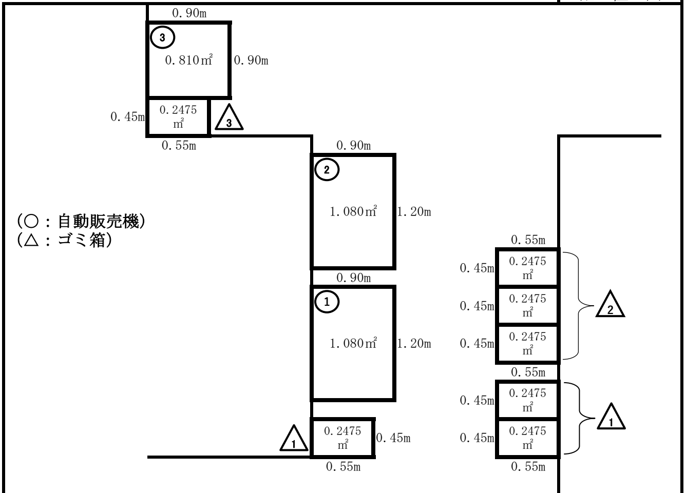
配置図
