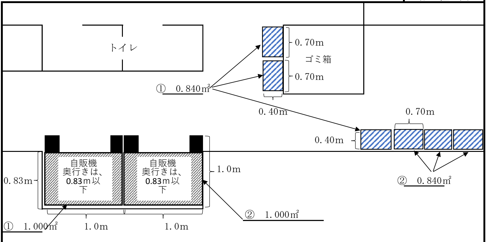
配置図
