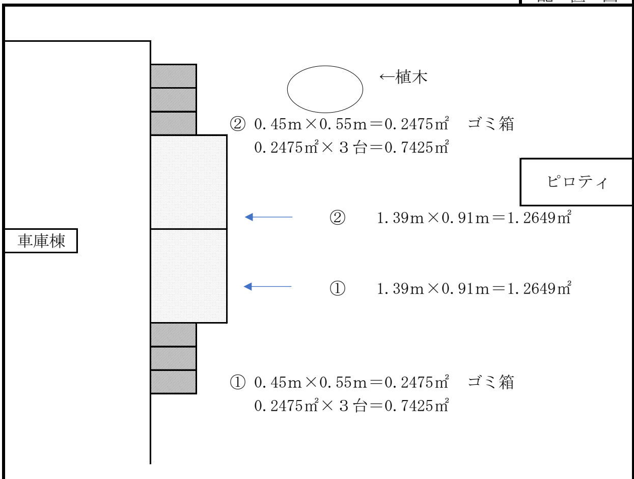
配 置 図
