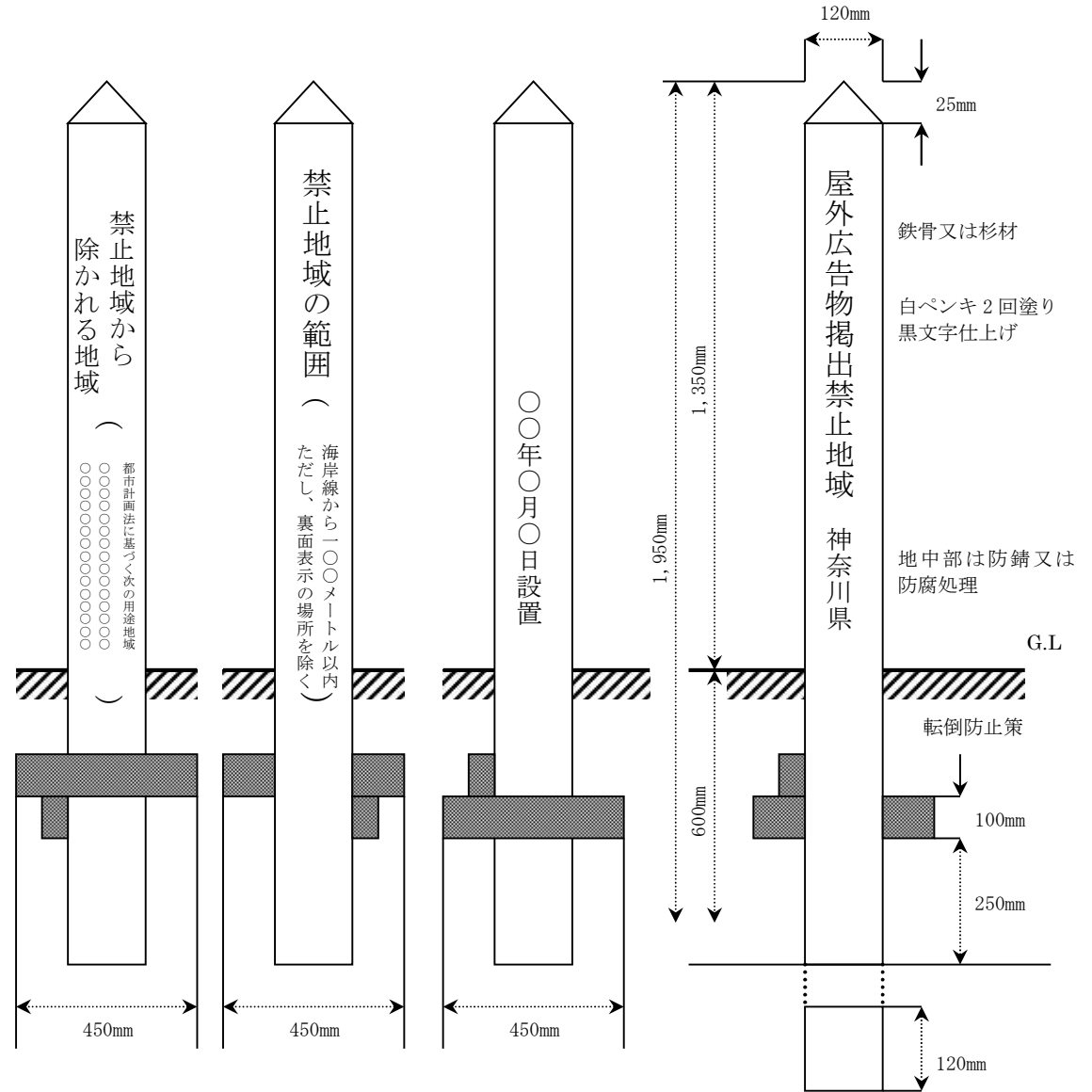
左側面図
