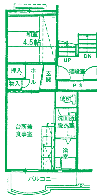
身体障害者向住宅 KN-6単 (車いす以外単身) (1DK)
