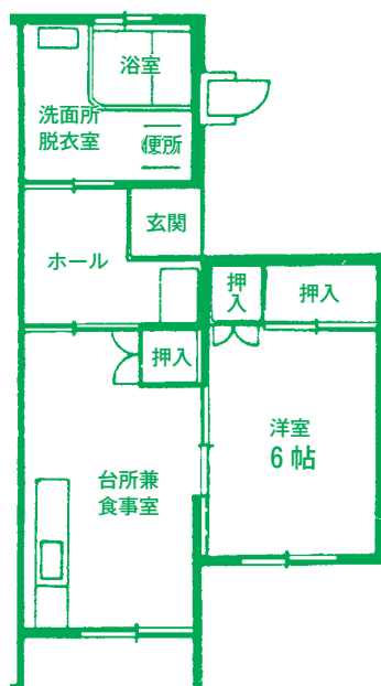
身体障害者向住宅 KFR-6単 (車いす単身) (1DK)
