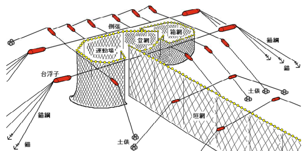
定置網の構造と各部の名称
