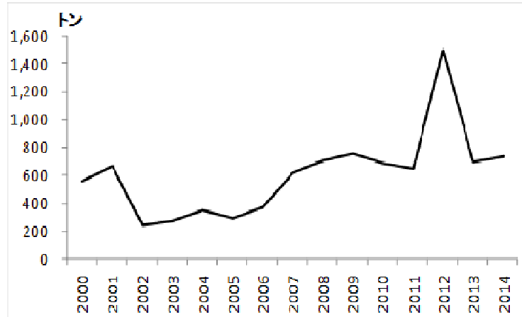
相模湾のブリ類漁獲量の経年変化 (定置網:2000~2014)
