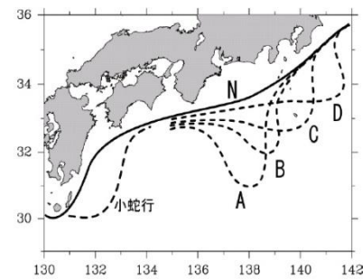
図1 黒潮流型の分類
