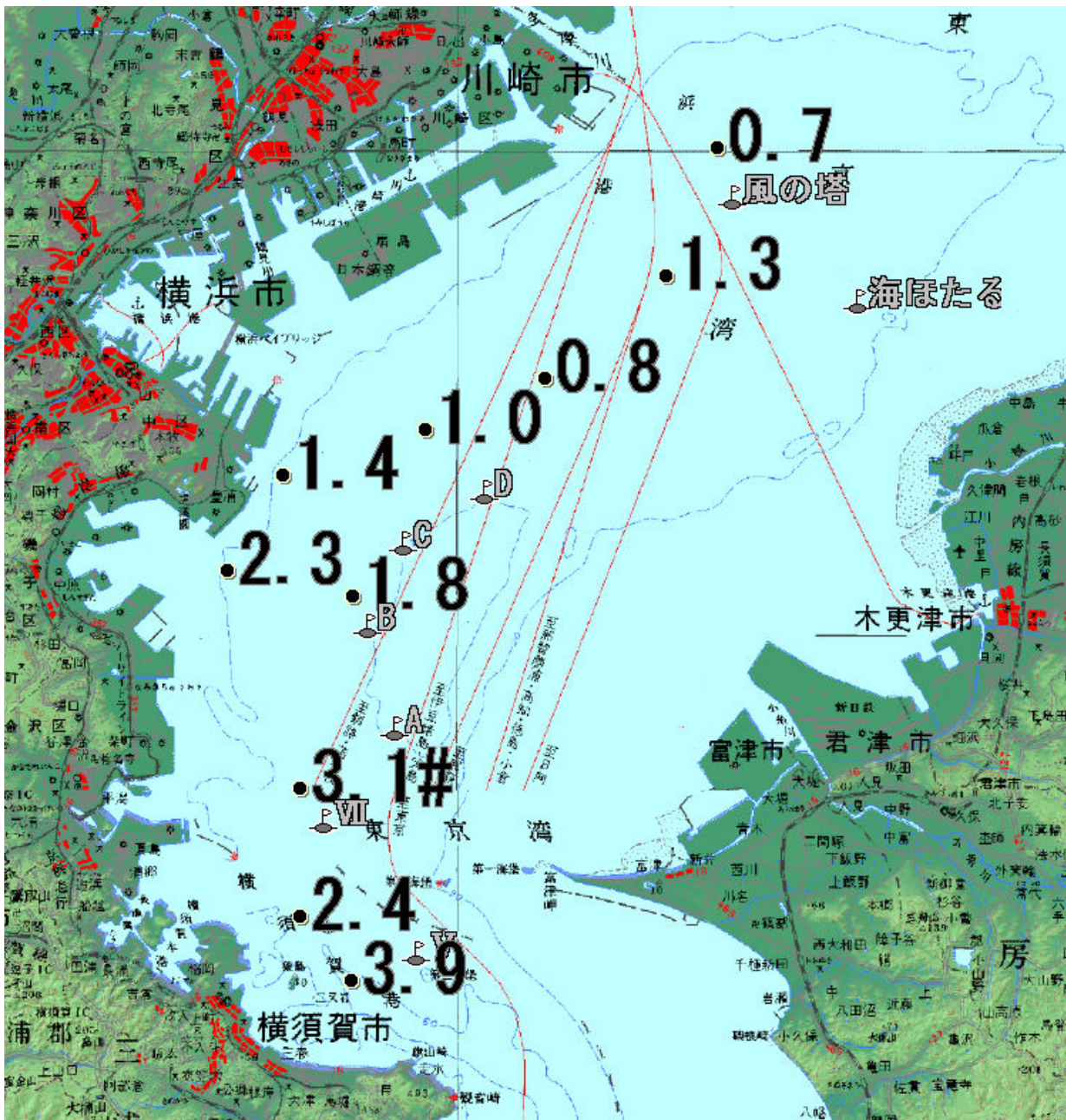
底層の溶存酸素量 (ml/l)
