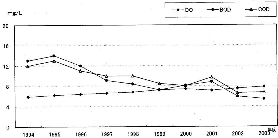
图3-6 境川(境橋)
