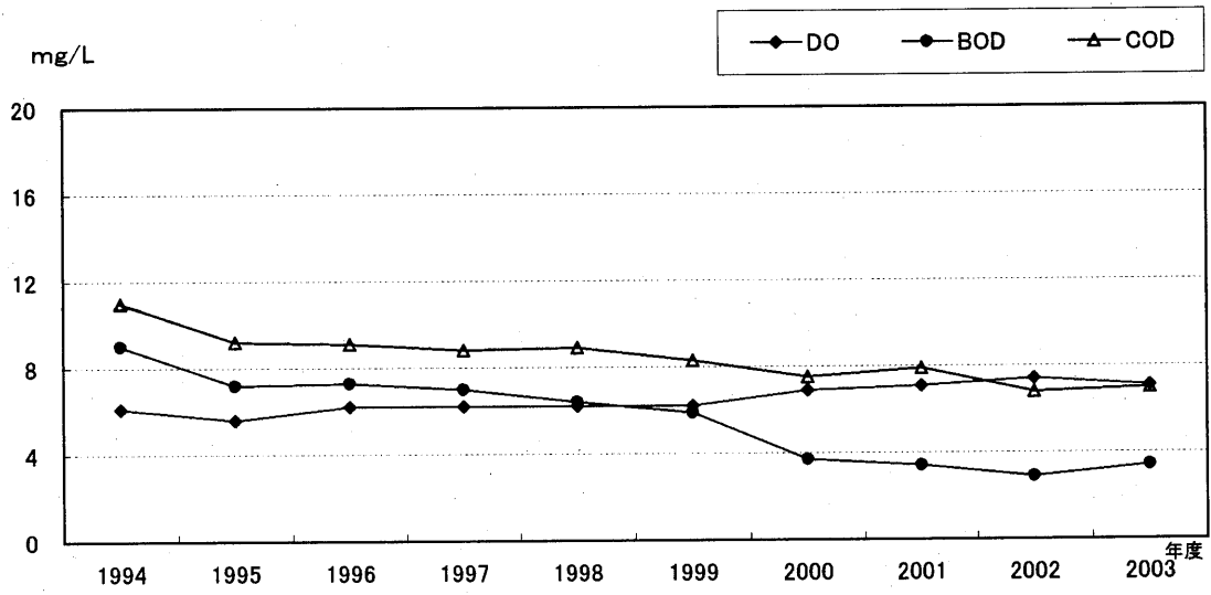
图3-5 境川(境川橋)
