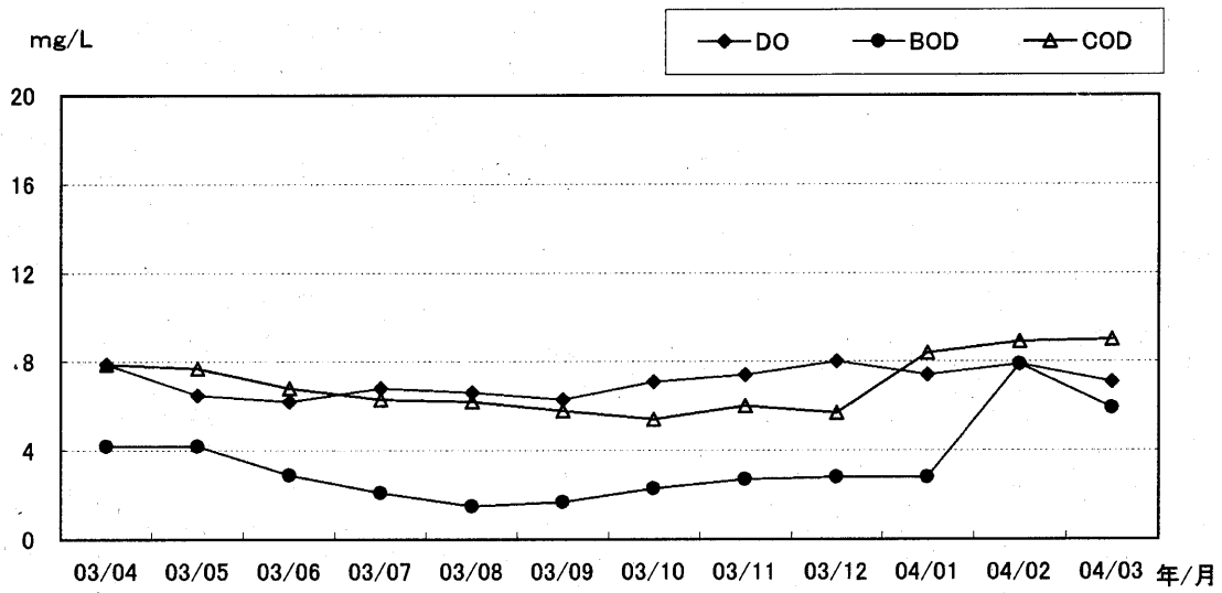
图4-5 境川(境川橋)
