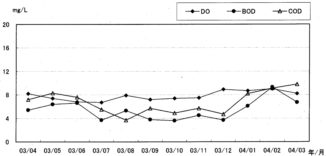
图4-6 境川(境橋)
