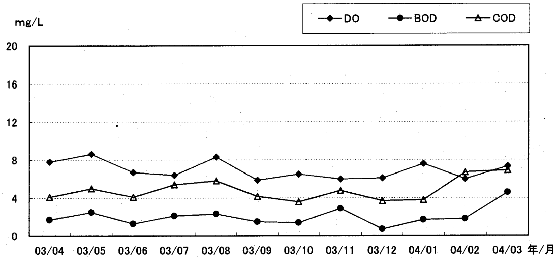
图4-5 境川(境川橋)
