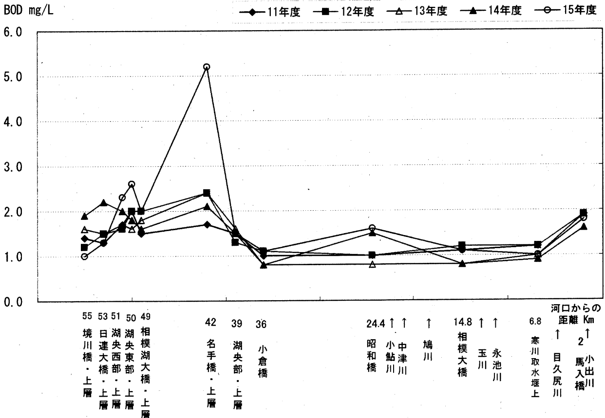
図2-4 相模川におけるBOD縦断変化図
