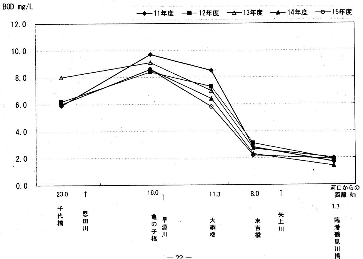
図2-2 鶴見川におけるBOD縦断変化図
