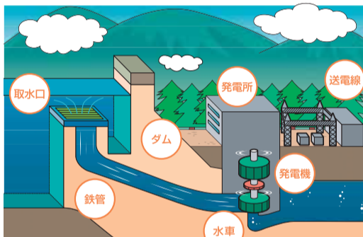
発電のしくみ(ダム式)
