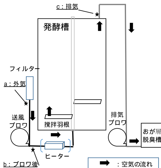
図 1 入排気温度・湿度と風量の測定箇所
