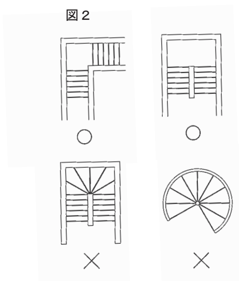
上段：設置が可能な階段の例 下段：設置が禁止される回り階段の例
