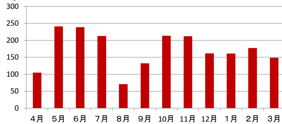
【kg】 桂川清流センターにおける全リンの負荷軽減量
