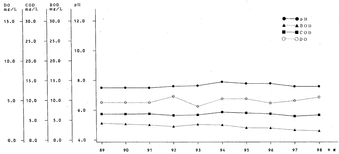
图3-5 境川 (境川橋)
