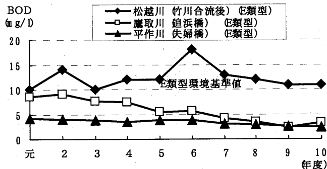
鷹取川、平作川、松越川のBOD年平均値の推移
