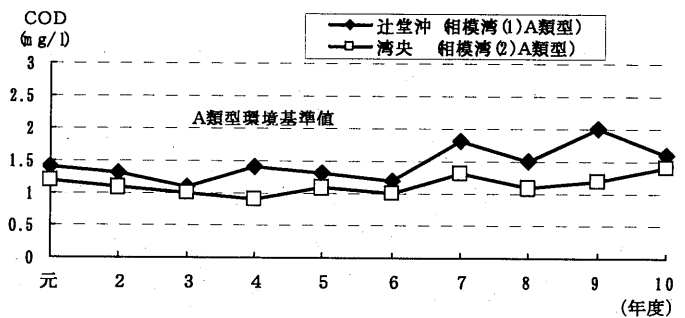
相模湾の主要地点におけるCOD年平均値の推移
