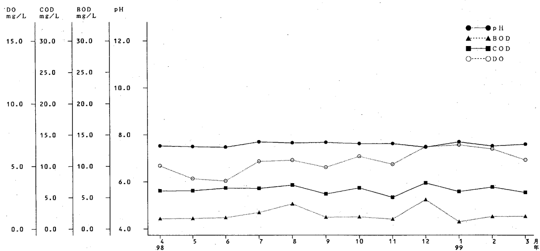
图 4-5 境川 (境川橋)
