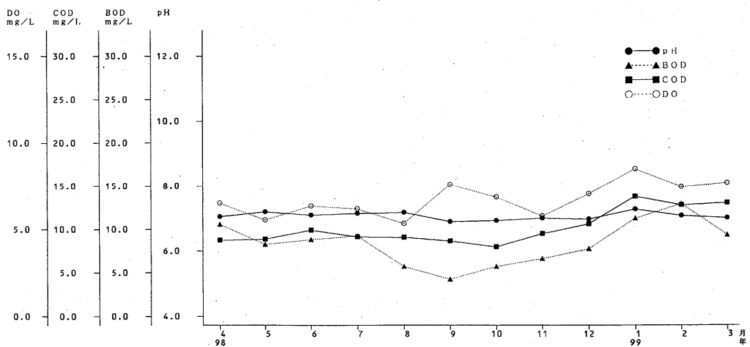
图 4-6 境川 (境橋)
