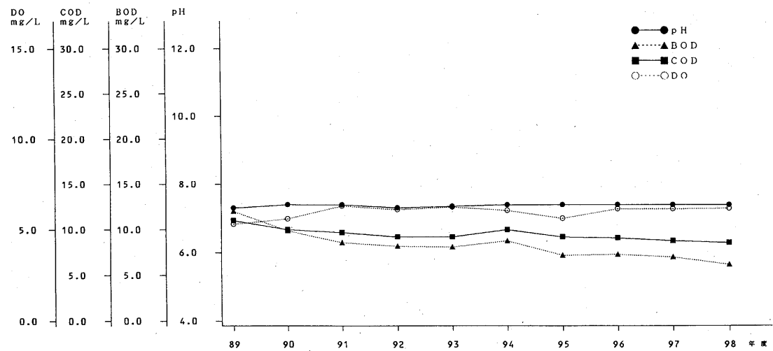
图3-6 境川 (境橋)
