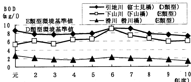
下山川、滑川、引地川におけるBOD年平均値の推移
