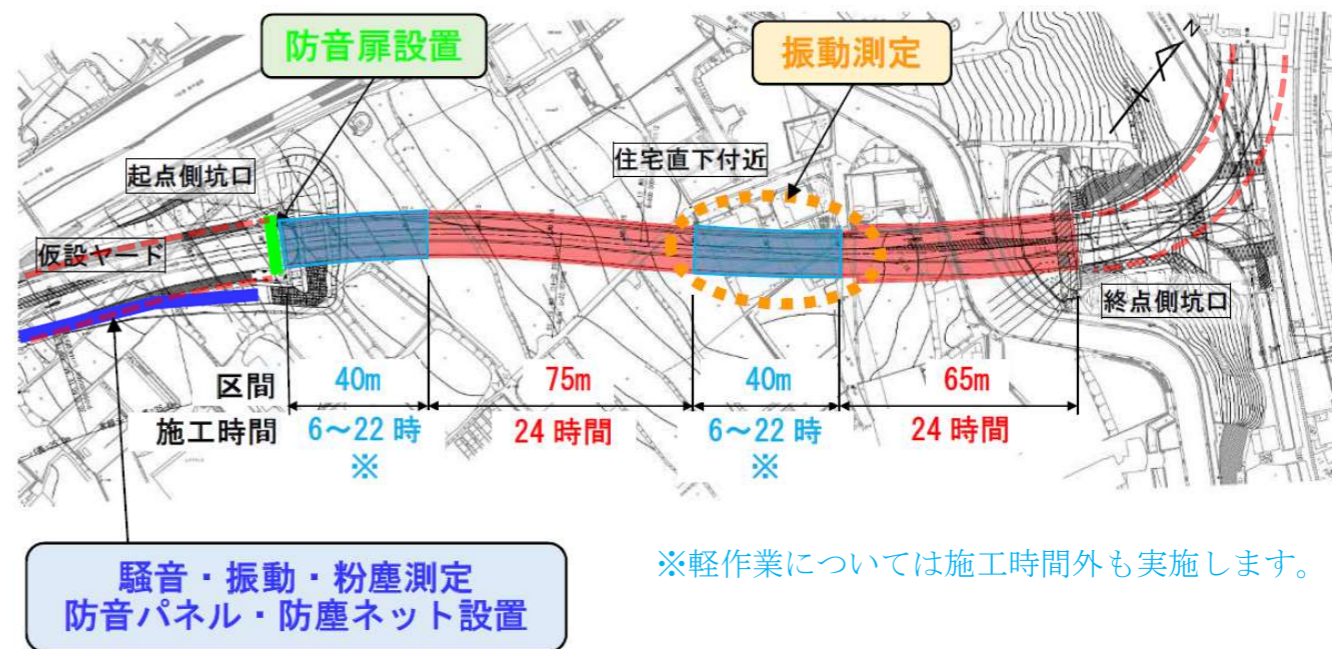
工事箇所拡大図
