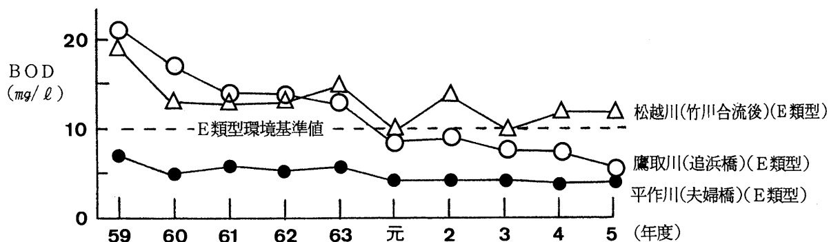
鷹取川、松越川、平作川におけるBOD年平均値の推移
