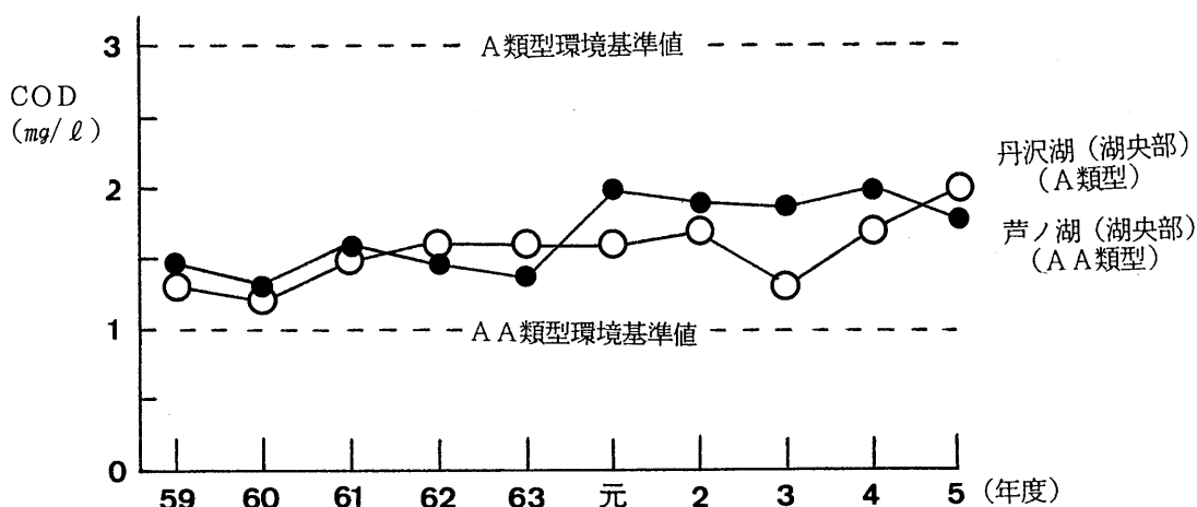
芦ノ湖、丹沢湖の主要地点におけるCOD年平均値の推移
