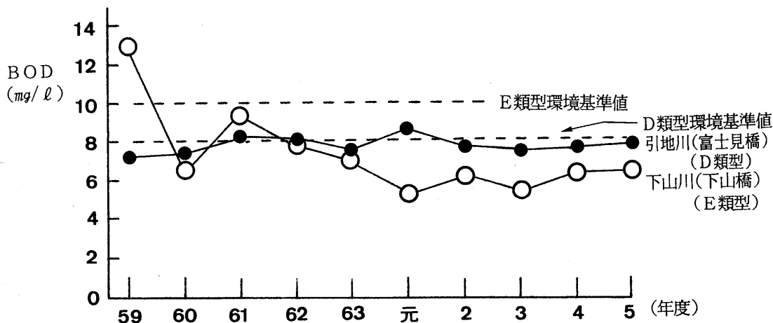
下山川、引地川におけるBOD年平均値の推移
