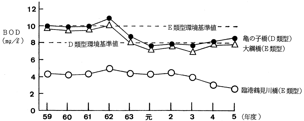
鶴見川主要地点におけるBODの年平均値の推移
