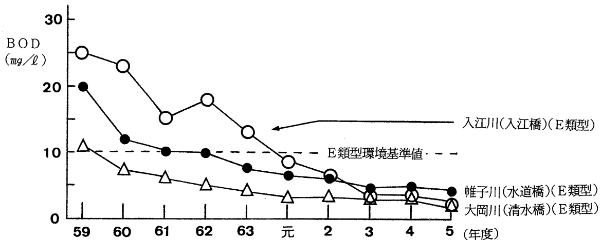
帷子川、大岡川、入江川におけるBOD年平均値の推移
