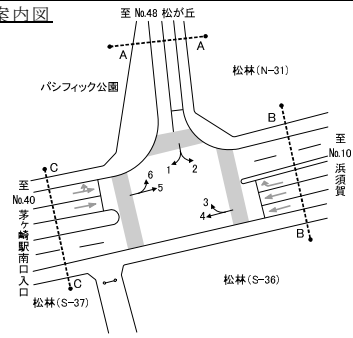
方向案内図
