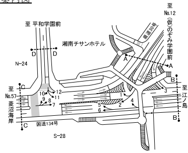
方向案内図
