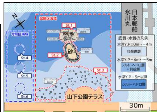
図2 平面図
