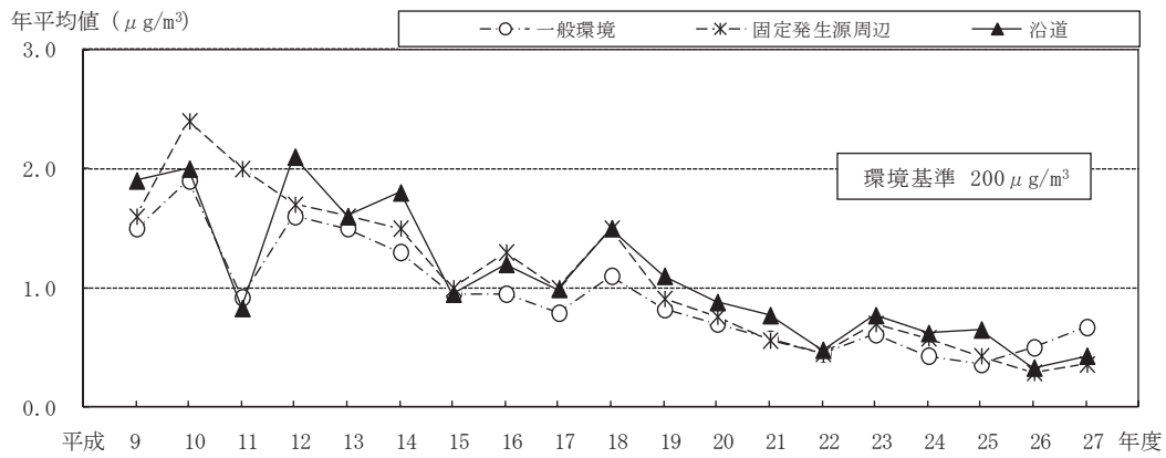
図 8-1-3 トリクロロエチレンの地域分類ごとの年平均値の経年推移
