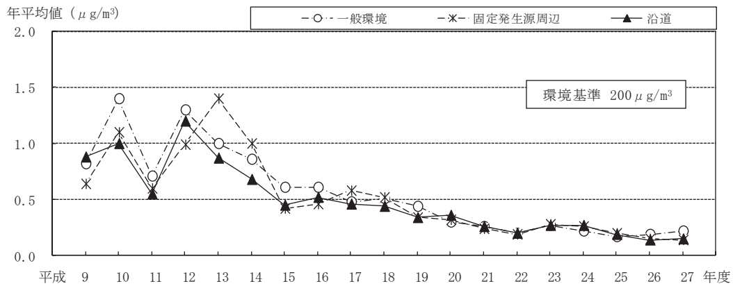
図 8-1-4 テトラクロロエチレンの地域分類ごとの年平均値の経年推移
