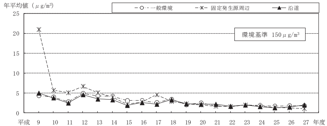
図 8-1-5 ジクロロメタンの地域分類ごとの年平均値の経年推移
