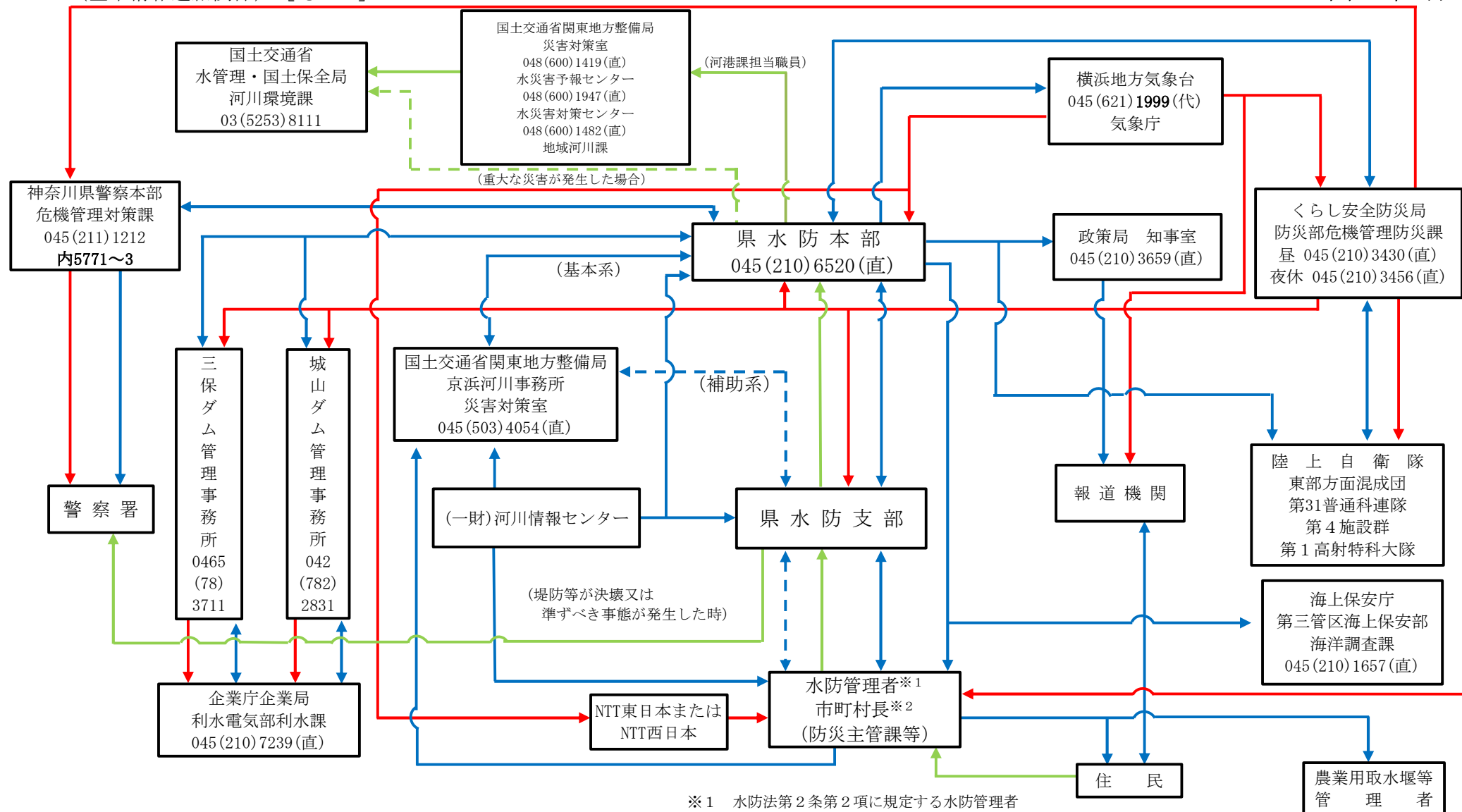
(3) 水防時における通信連絡基本系統図 (基本情報連絡関係) [その1]
