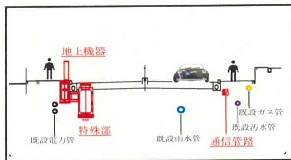
(計画横断面)
