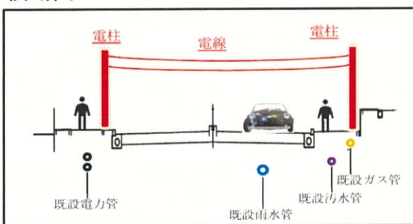
(現況横断面)
