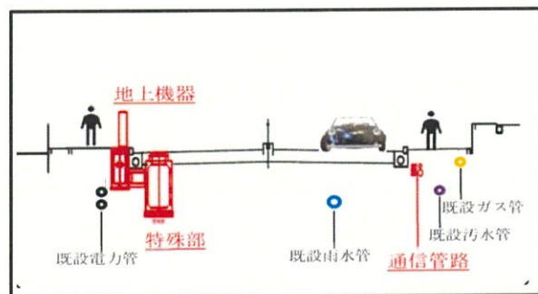
(計画横断面)
