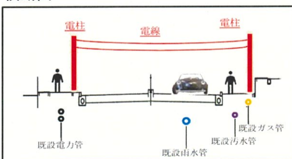
(現況横断面)
