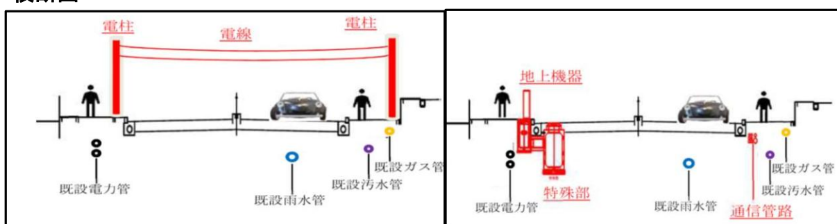
(現況横断面図)
