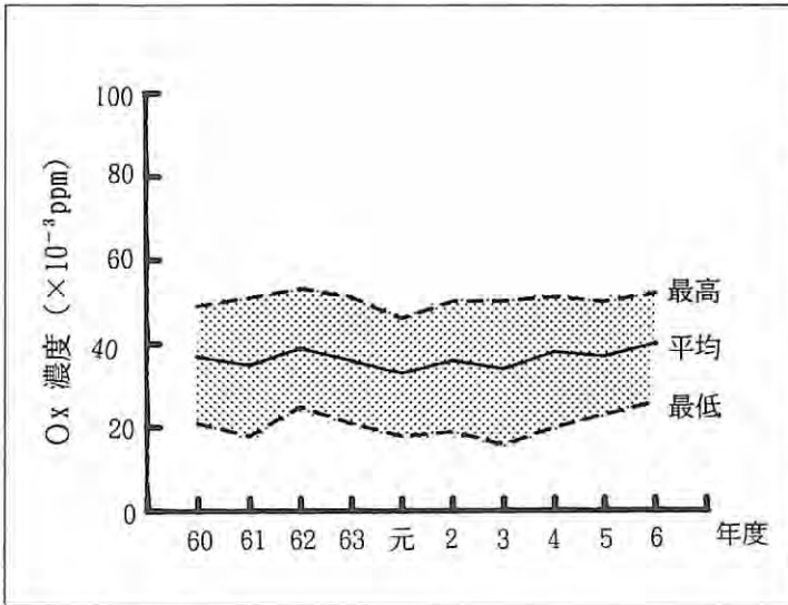
図は、Ox濃度の昼間の局別日最高1時間値の月平均値から月ごとに求めた一般環境大気測定局の平均値、最大値、最低値を示す。
