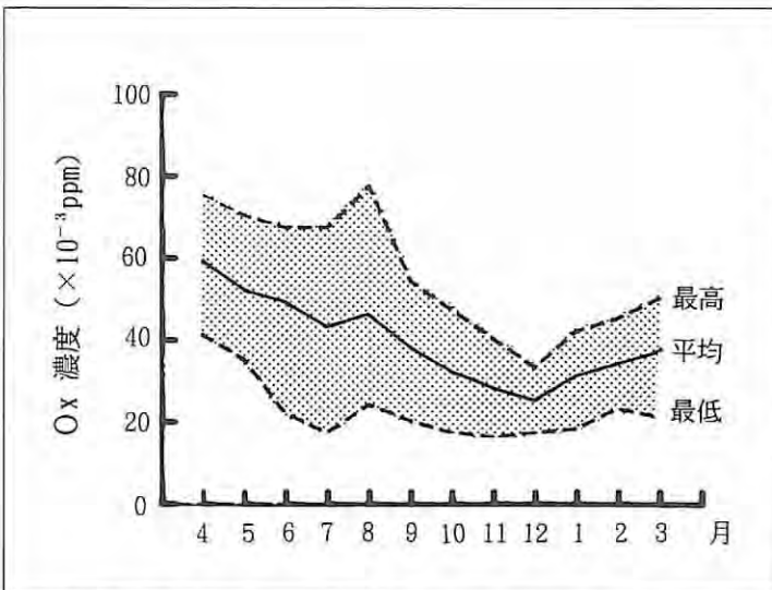
図は、各測定局におけるOxの昼間の日最高1時間値の年平均値から求めた一般環境大気測定局の平均値、最大値、最低値を示す。
