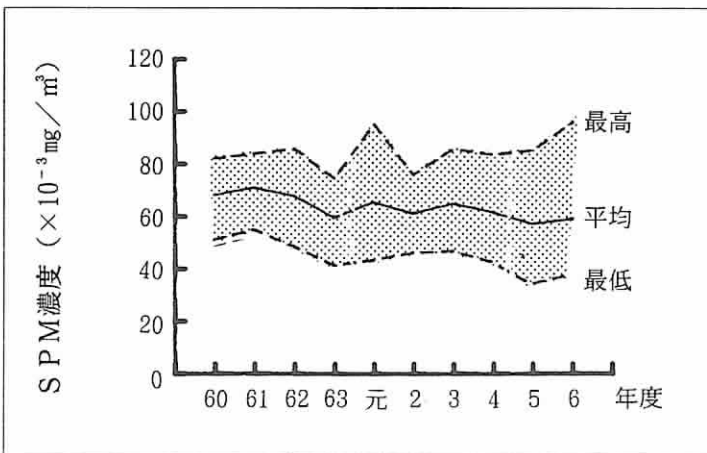
図は、各測定局におけるSPMの年平均値から年度ごとに求めた自動車排出ガス測定局の平均値、最大値、最低値を示す。
