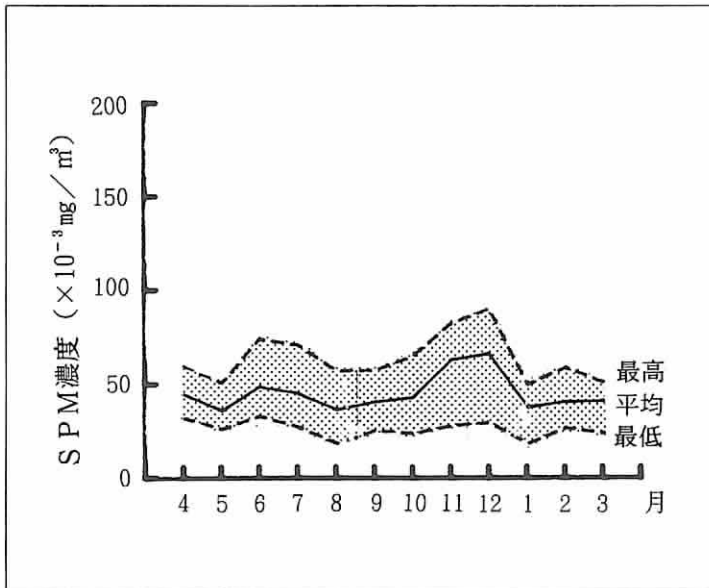
図は、一般環境大気測定局におけるSPMの月平均値から月ごとに求めた平均値、最大値、最低値を示す。
