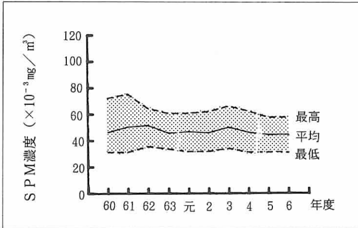
図は、各測定局におけるSPMの年平均値から年度ごとに求めた一般環境大気測定局の平均値、最大値、最低値を示す。
