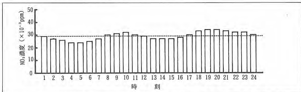
図は、NO 2 濃度の年間測定結果から時間帯別に求めた一般環境大気測定局の平均値を示す。NO 2 濃度の時刻変化は、午前8時から11時と午後5時以降が高い二山型となっている。
