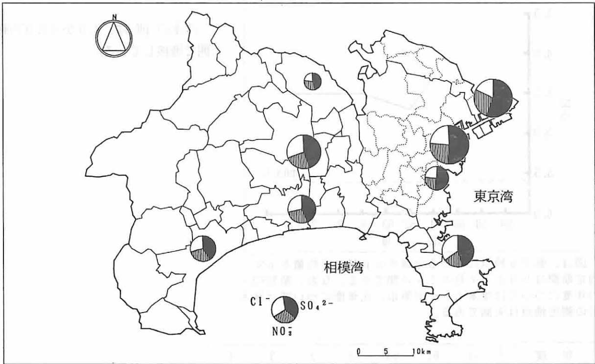
図は、県下8地点における全降水の SO_4^{2-} 、 NO_3^- 、 Cl^- 濃度から求めた各成分の当量濃度の割合を示す。また、円の面積は3成分の当量濃度の合計量を表す。なお、測定期間は、6月から7月の2カ月間である。
