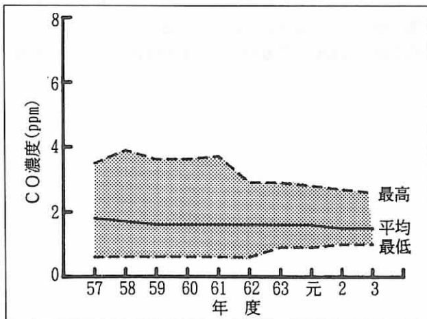
図は、各測定局におけるCOの年平均値から年度ごとに求めた自動車排出ガス測定局の平均値、最大値、最小値を示す。
