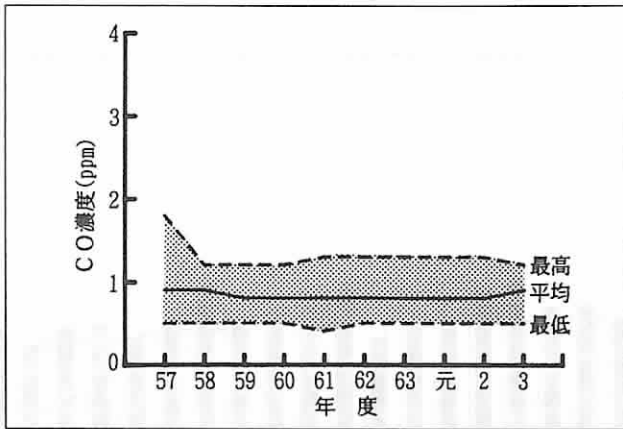
図は、各測定局におけるCOの年平均値から年度ごとに求めた一般環境大気測定局の平均値、最大値、最小値を示す。
