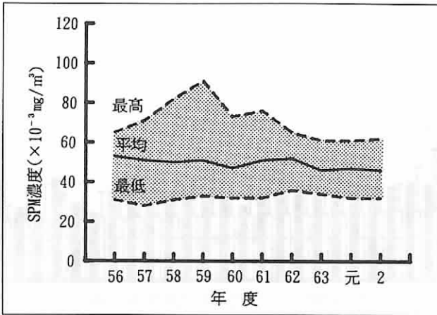
図は、各測定局におけるSPMの年平均値から年度ごとに求めた一般環境大気測定局の平均値、最大値、最小値を示す。
