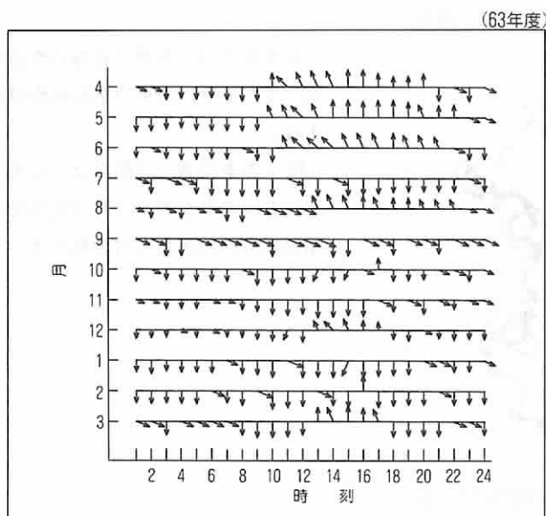
図は、厚木市役所における風向風速の観測結果から求めた月別時刻別の最多風向及び平均風速を示す。
