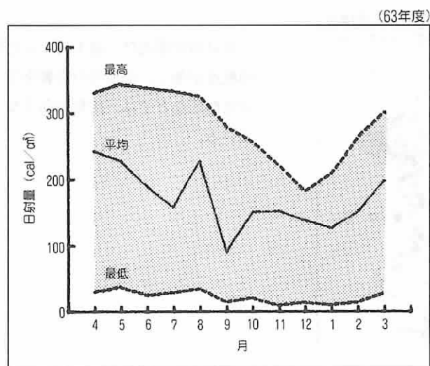
図は、横浜市中区本牧の12時における日射量の月ごとに求めた平均値、最高値、最低値を示す。
