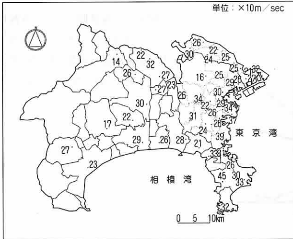
図は、実測した風速の年平均値から求めた高度20mに相当する年間平均風速の地域分布を示す。
