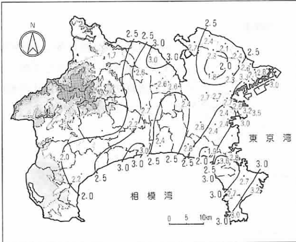
図は、実測した風速の年間平均値から求めた、高度20mに相当する年平均風速の地域分布を示す。
