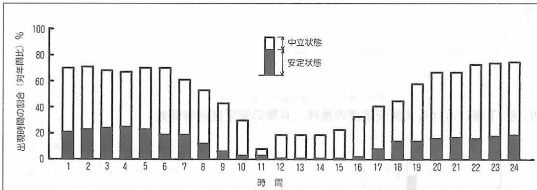
図は、横浜市中区にあるマリントワー〔78〕において毎時間観測している垂直方向の温度差の測定結果から月ごとに求めた、大気の安定状態及び中立状態の出現割合を示す。安定状態及び中立状態とは、地上78mと22mの温度差(78mの温度-22mの温度)から換算した100mあたりの気温減率 x が x \geq -0.6^{\circ}\text{C} (安定)と -0.6^{\circ}\text{C} > x \geq -1.0^{\circ}\text{C} (中立)である状態を示す。
