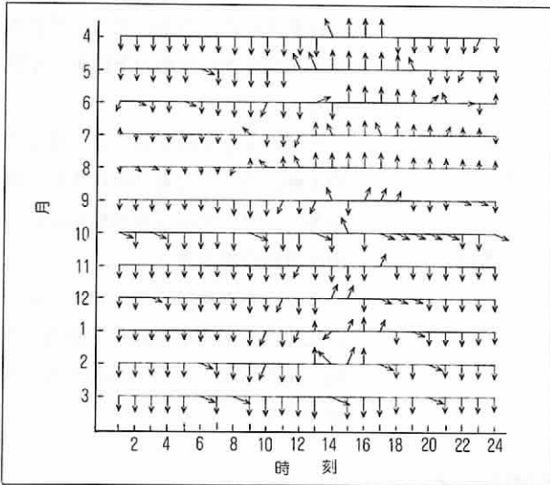
図は、厚木市役所〔67〕における風向風速の観測結果から求めた、月・時刻別の最多風向及び平均風速を示す。
