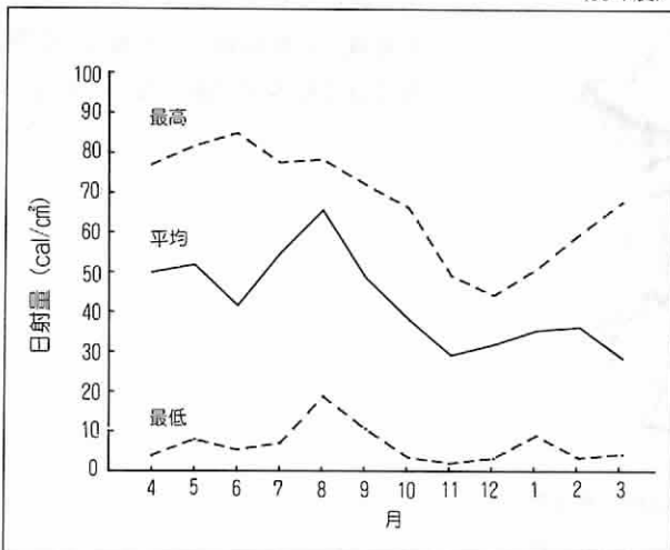
図は、横浜市中区本牧〔28〕の12時間における日射量の月ごとに求めた、平均値、最高値、最低値を示す。
