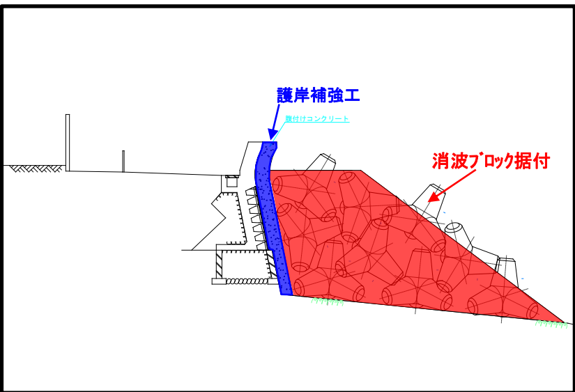
護岸補強工
